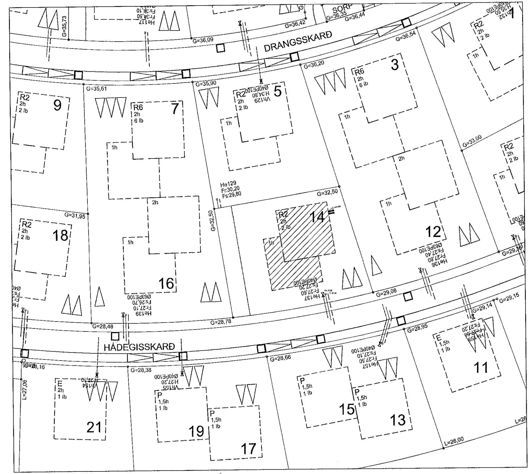
Afstöðumynd 1:500
