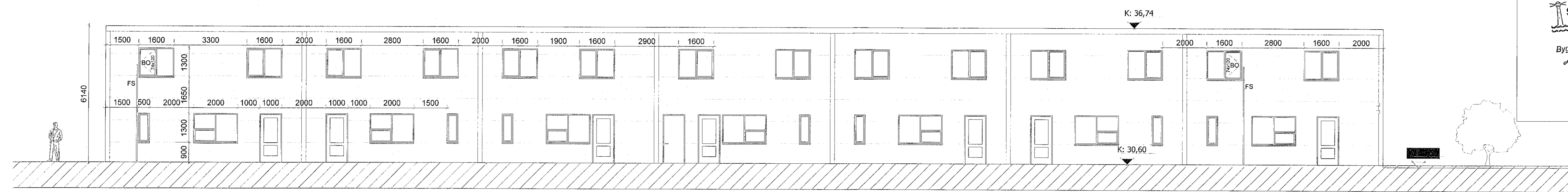
ÚTLIT AUSTUR 1:100
