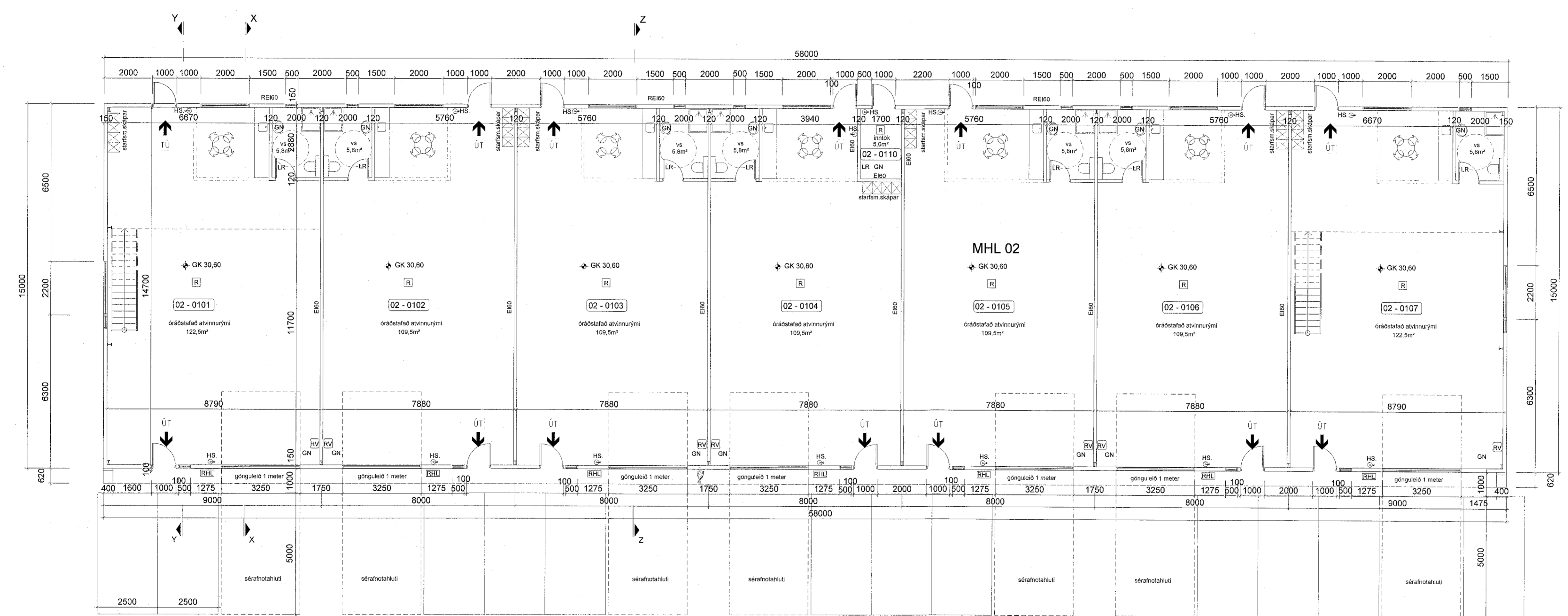
GRUNNMYND 1:100
