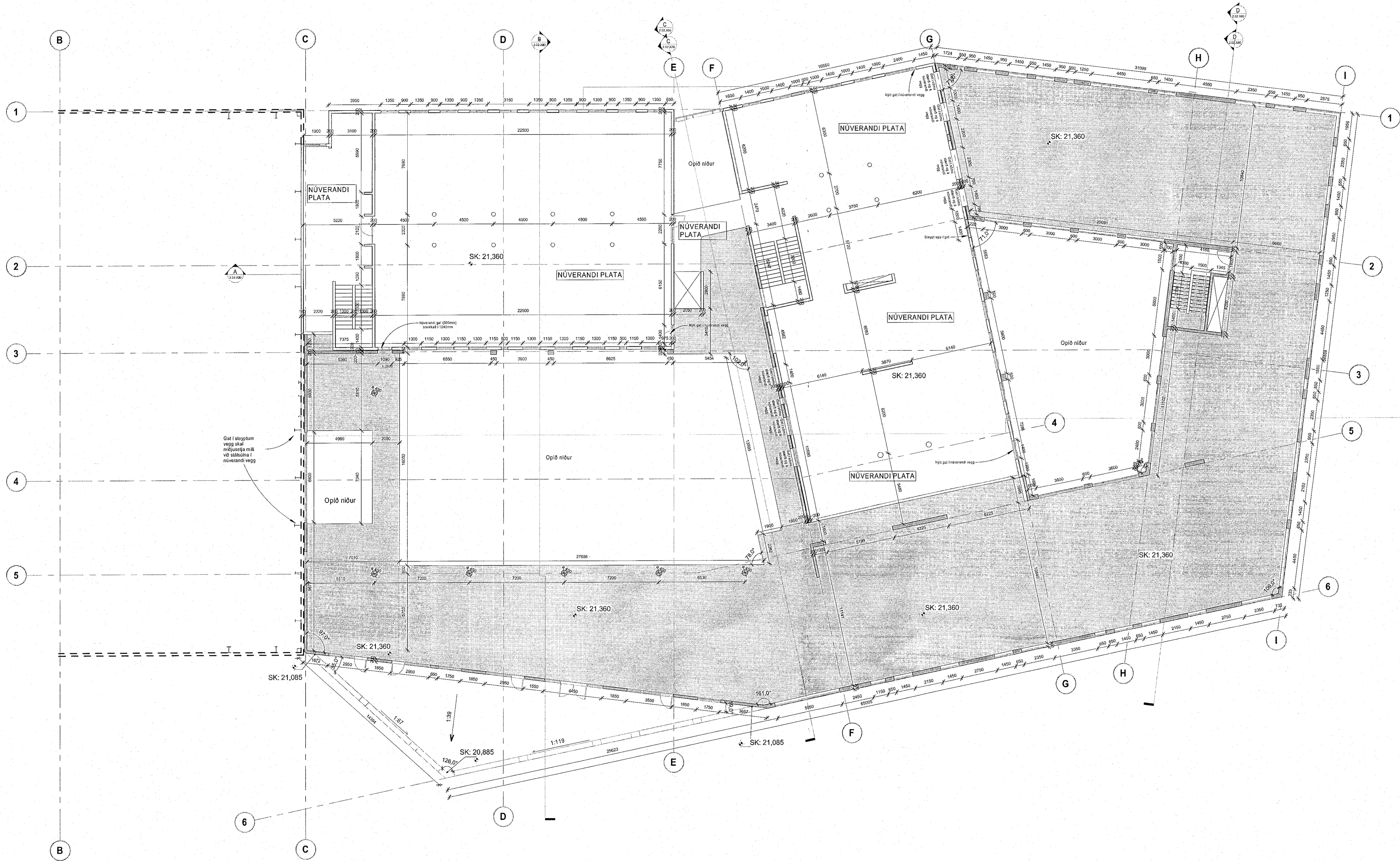
Hæð 3 STEYPA_yfirlit 1:150
