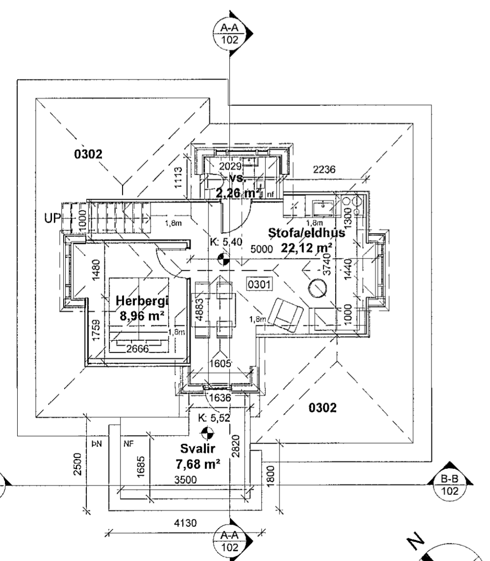
3 3. hæð 1 : 100
