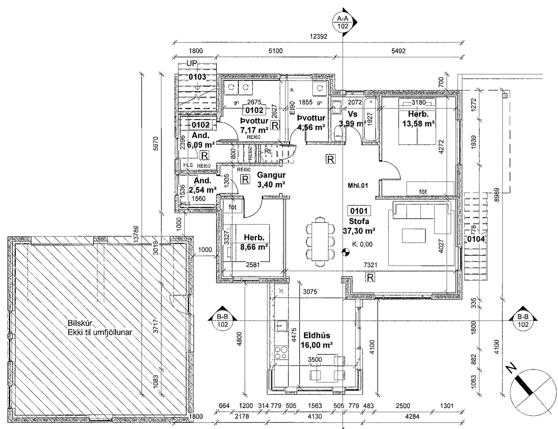
1 1. Hæð 1 : 100
