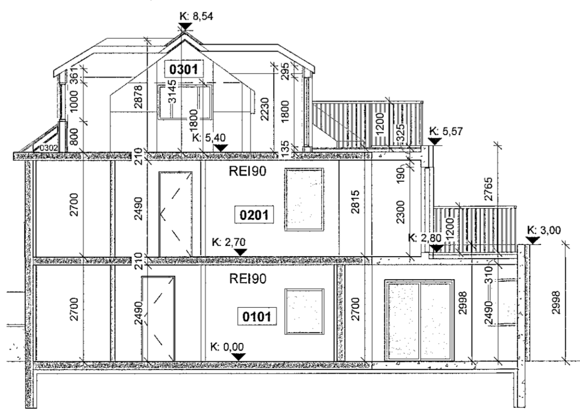
A-A Snið A-A 1 : 100
