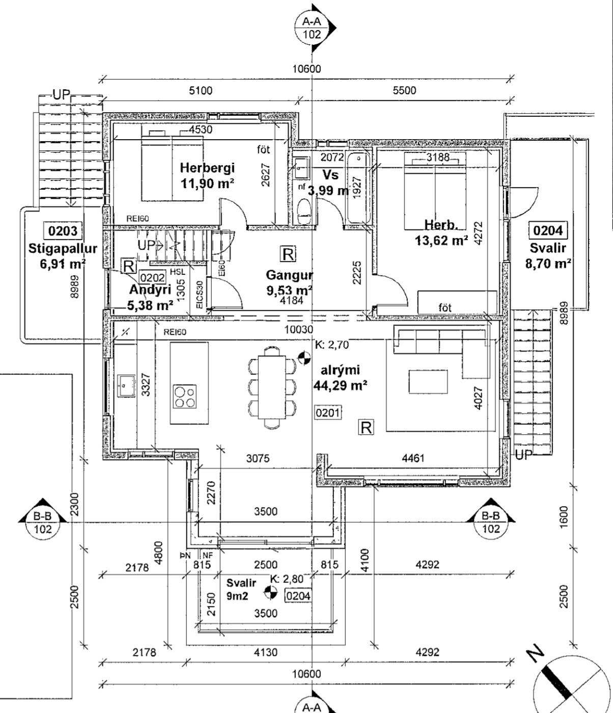
2 2. Hæð 1 : 100
