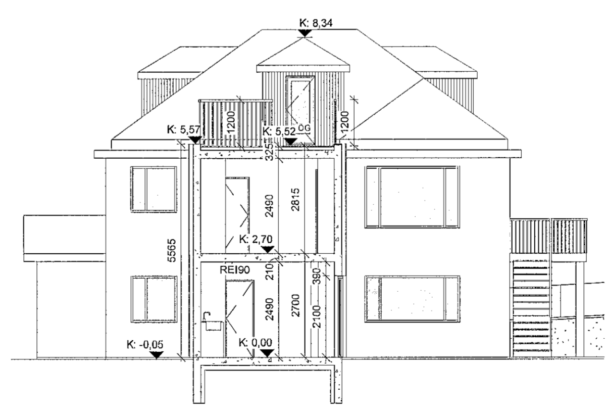
B-B Snið B-B 1 : 100
