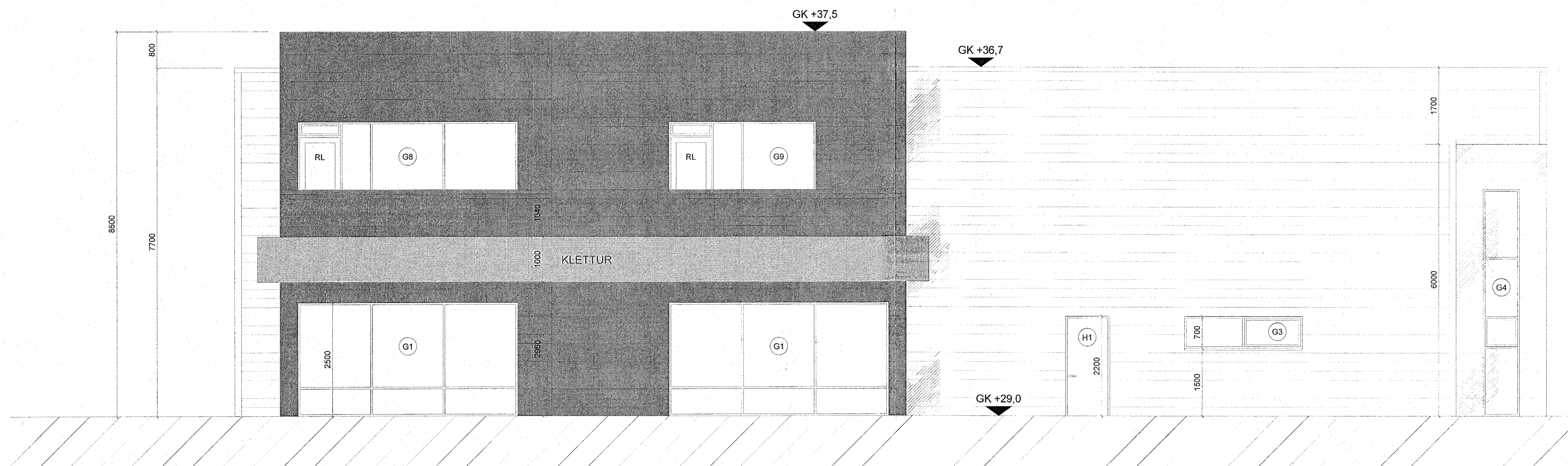
ÚTLIT VESTUR 1:50
