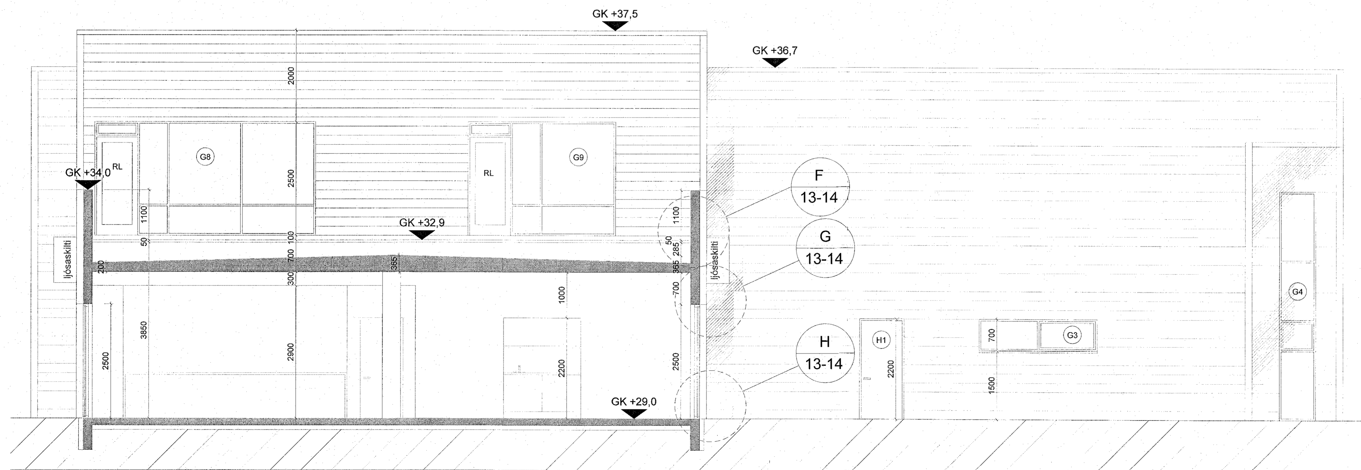
SNEIDING Æ-Æ 1:50
