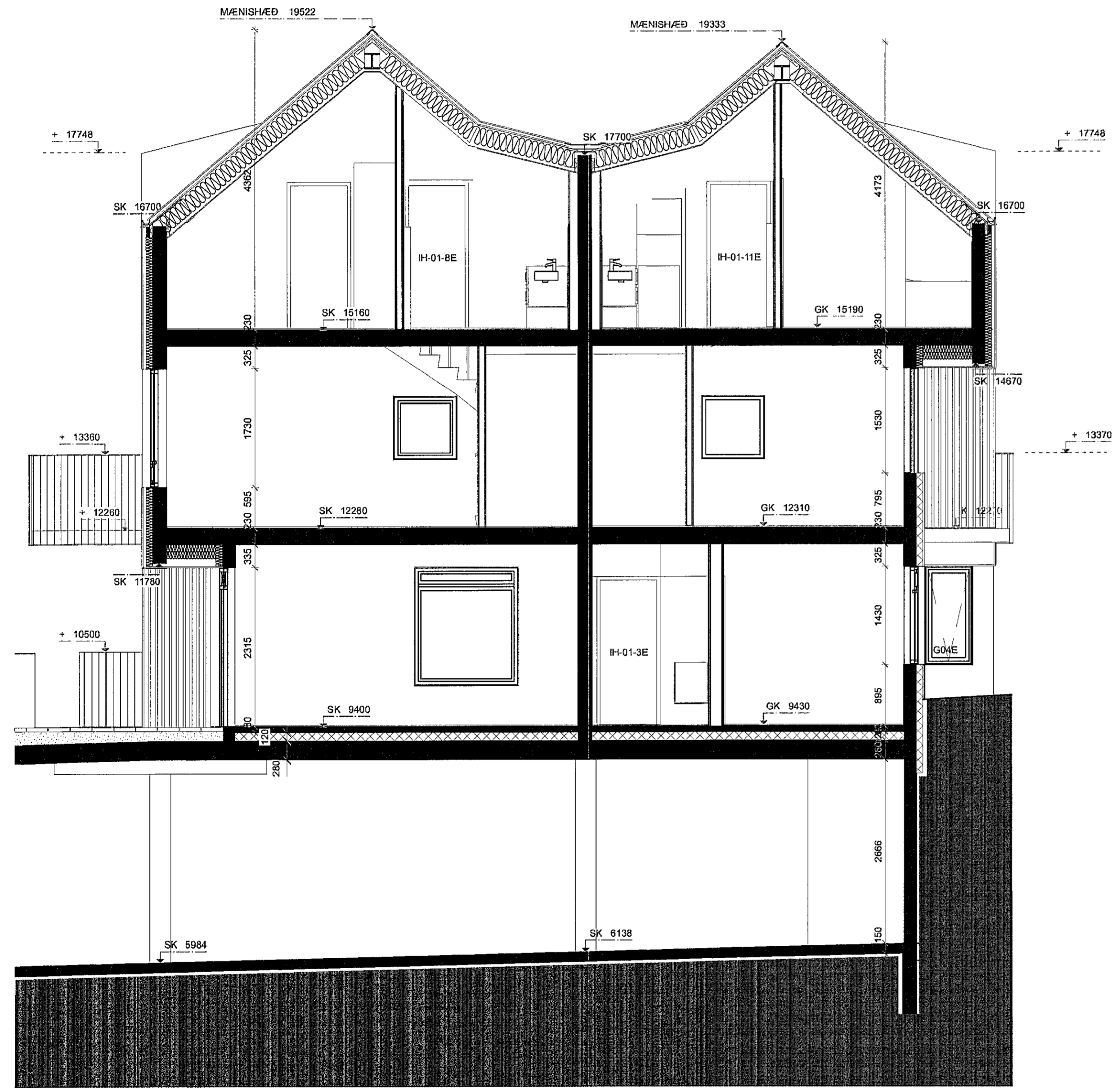
E3 SNEIÐING E3 Skali: 1:50
