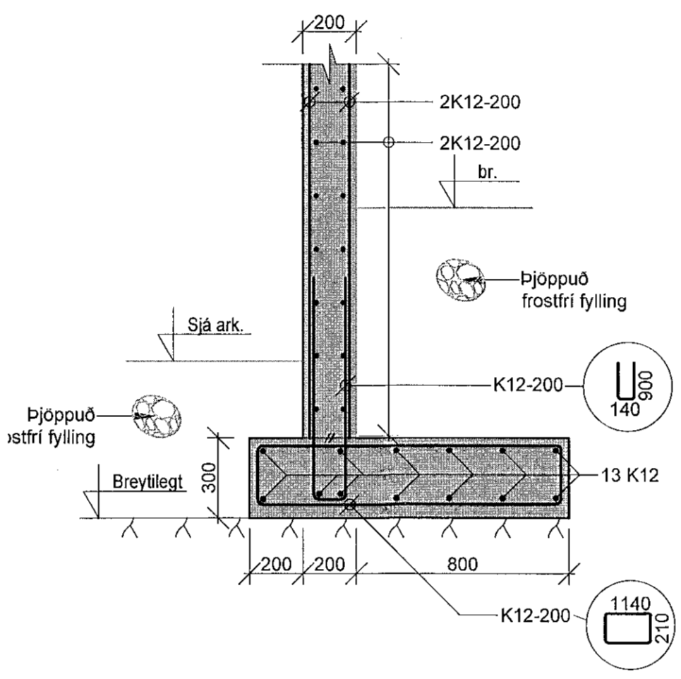
AG Snið M 1:20
