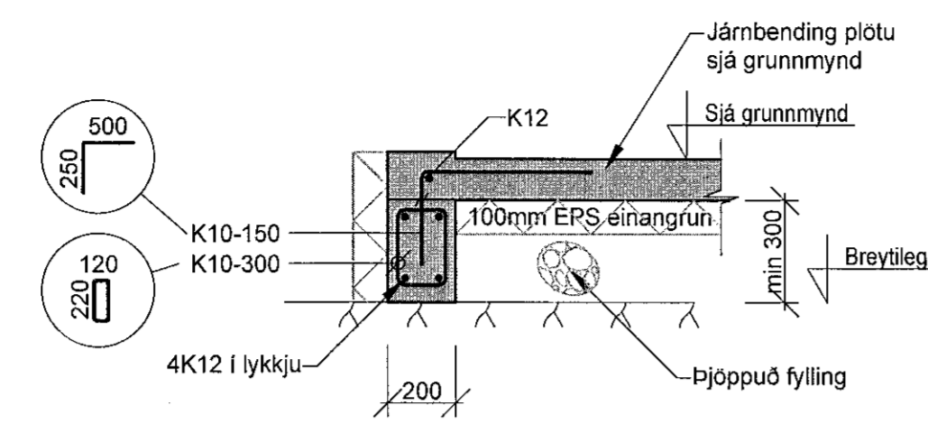
AB Snið M 1:20
