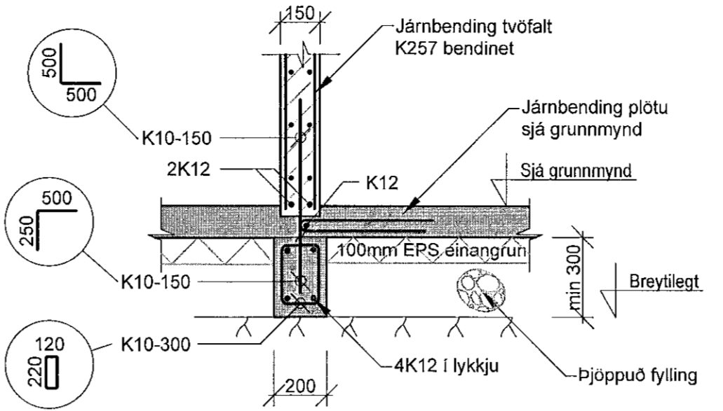
AC Snið M 1:20
