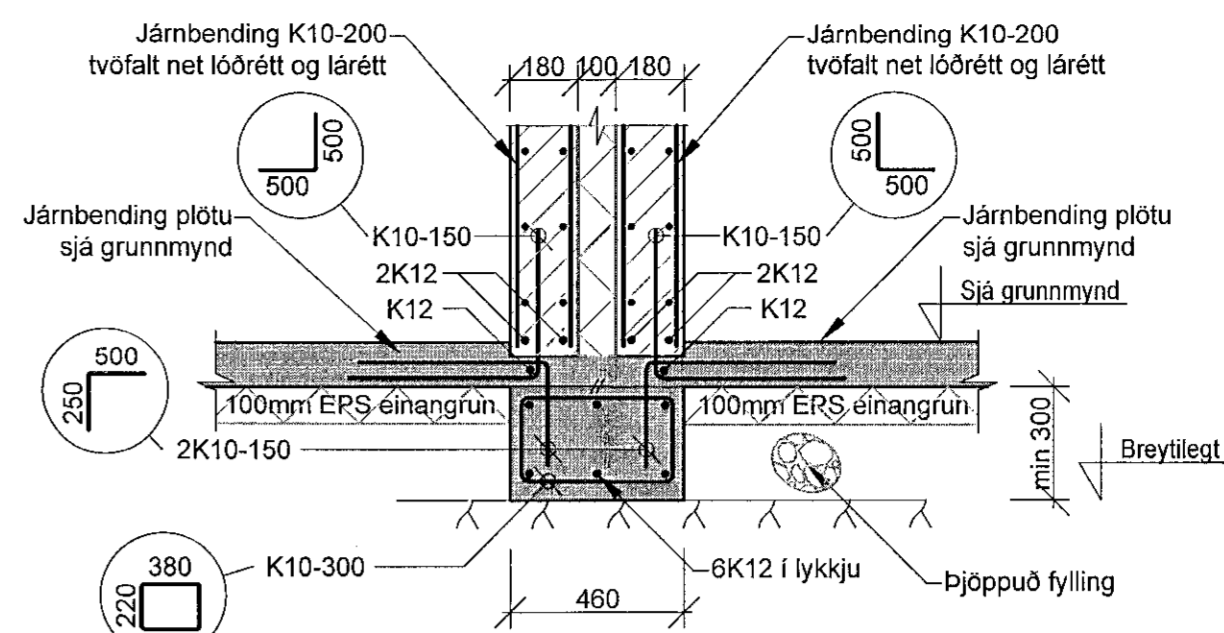
AD Snið M 1:20
