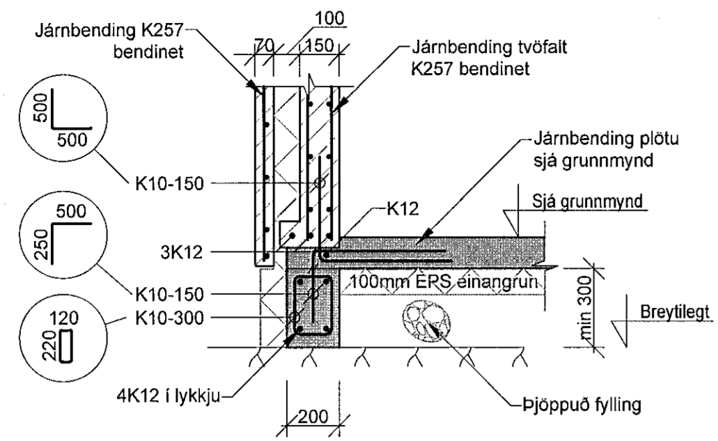
AA Snið M 1:20
