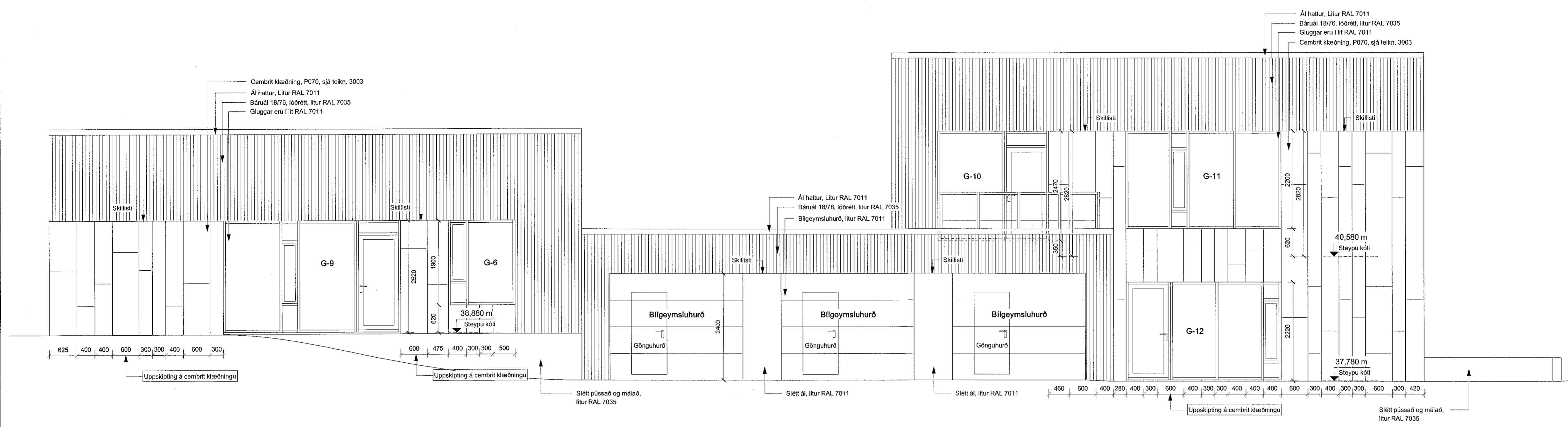
VERKT. - ÁSÝND SUÐUR mkv: 1 : 50
