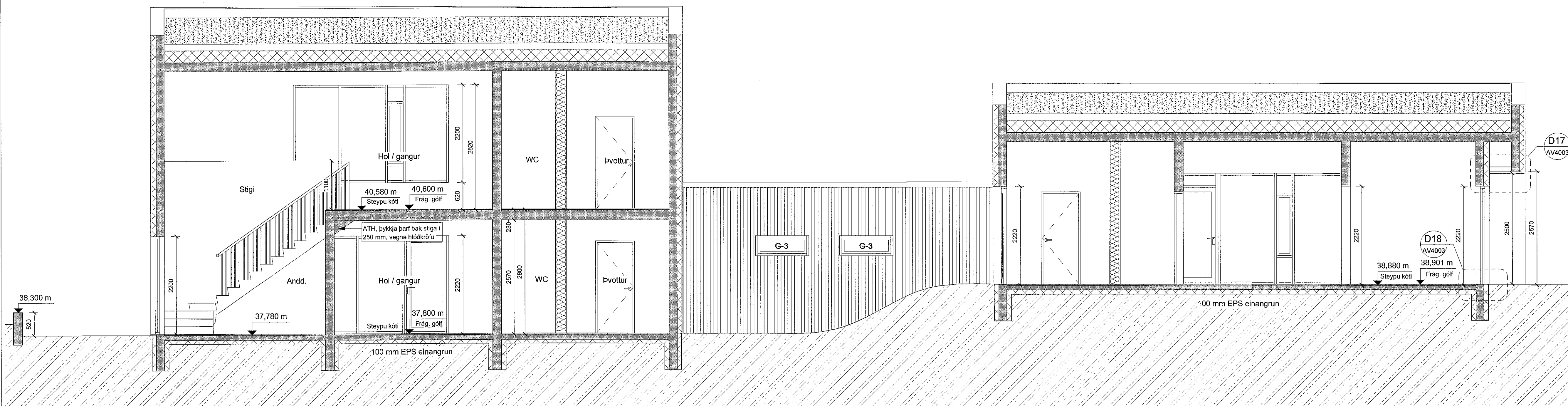
VERKT. SNID B-B mkv: 1 : 50
