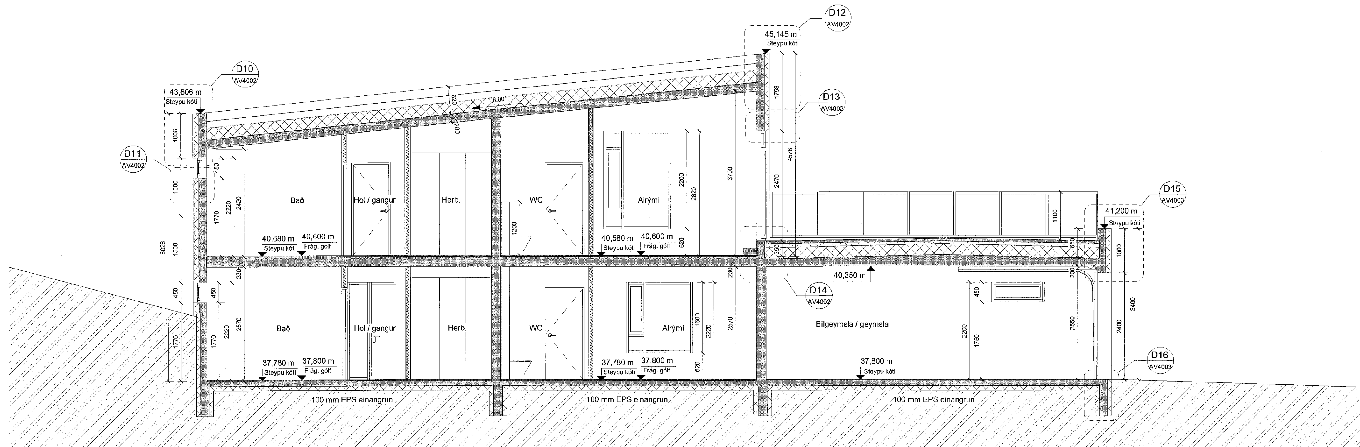
VERKT. SNID A-A mkv: 1 : 50
