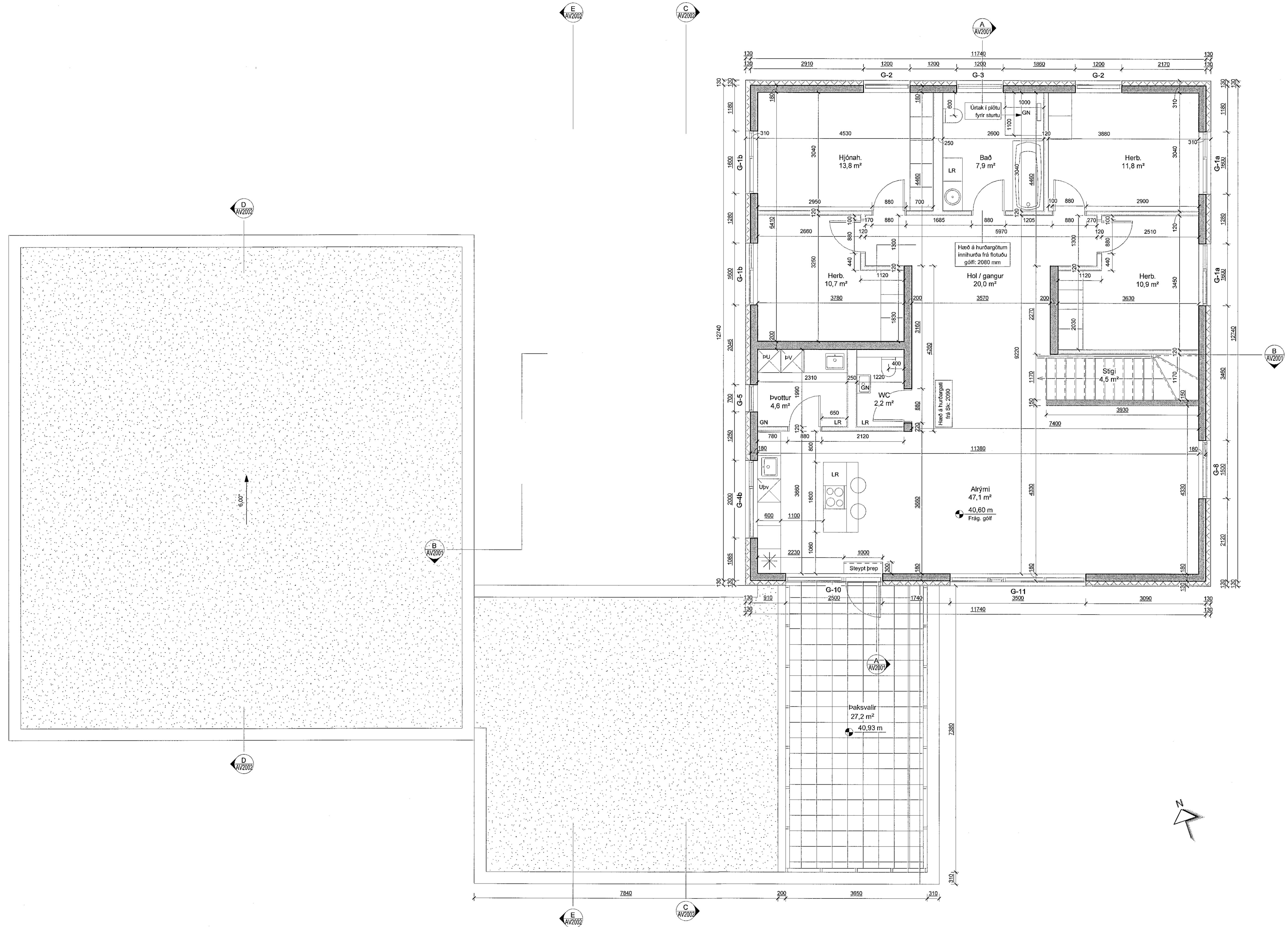
VERKT. GRUNNMYND 2. HÆÐ mkv: 1 : 50
