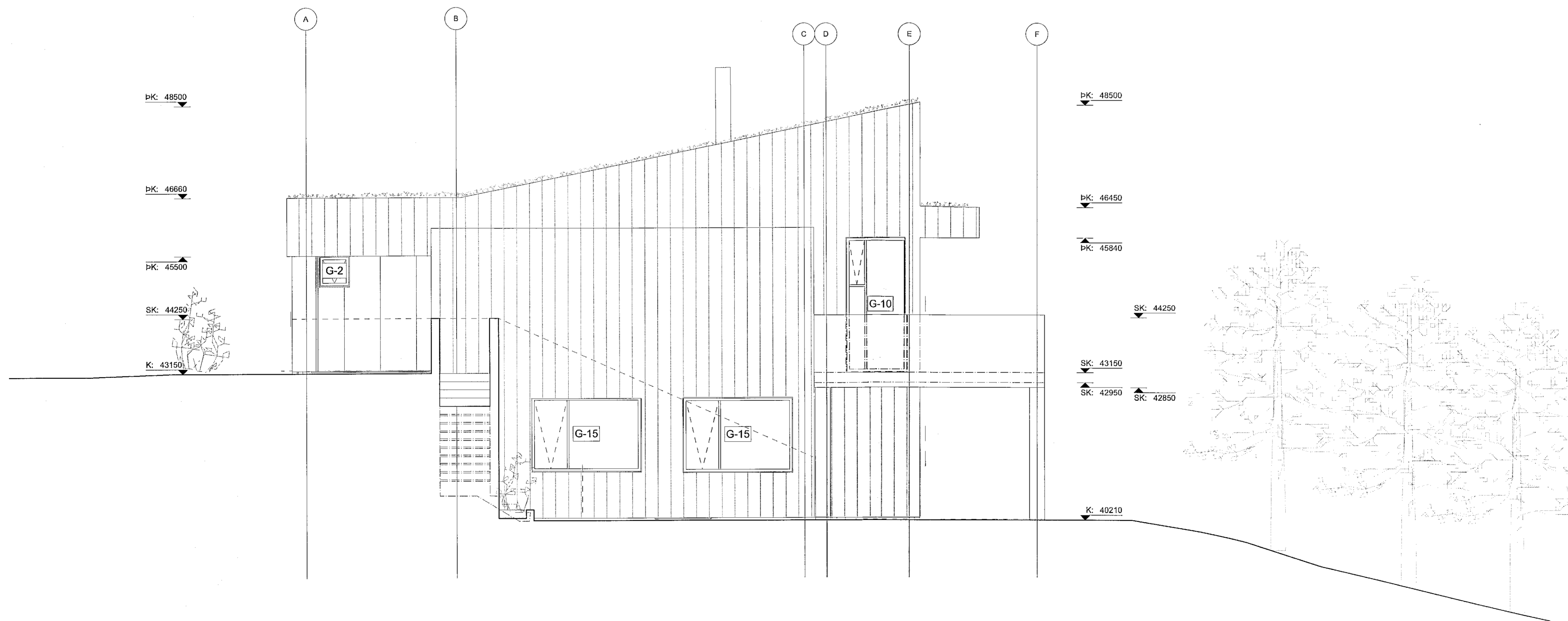
Ásýnd norðvestur mkv: 1:50 - A1 / 1:100 - A3
