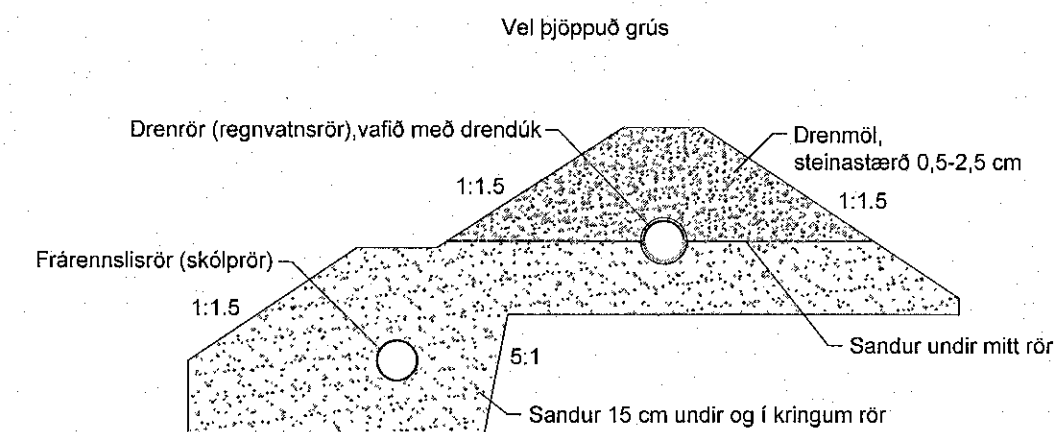
Frágangur röra 1:20
