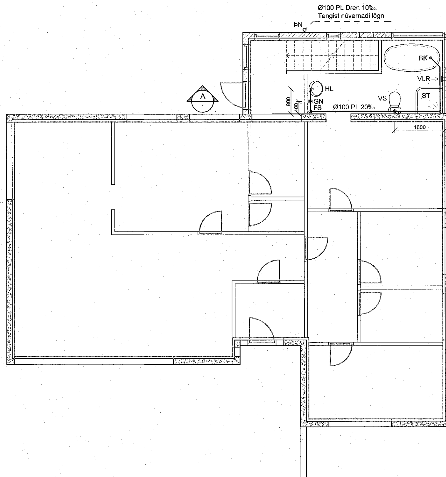
Grunnmynd efri hæð, frárennsli 1:50
