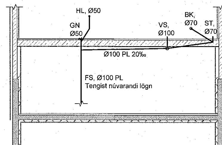
A Snið 1 1:50
