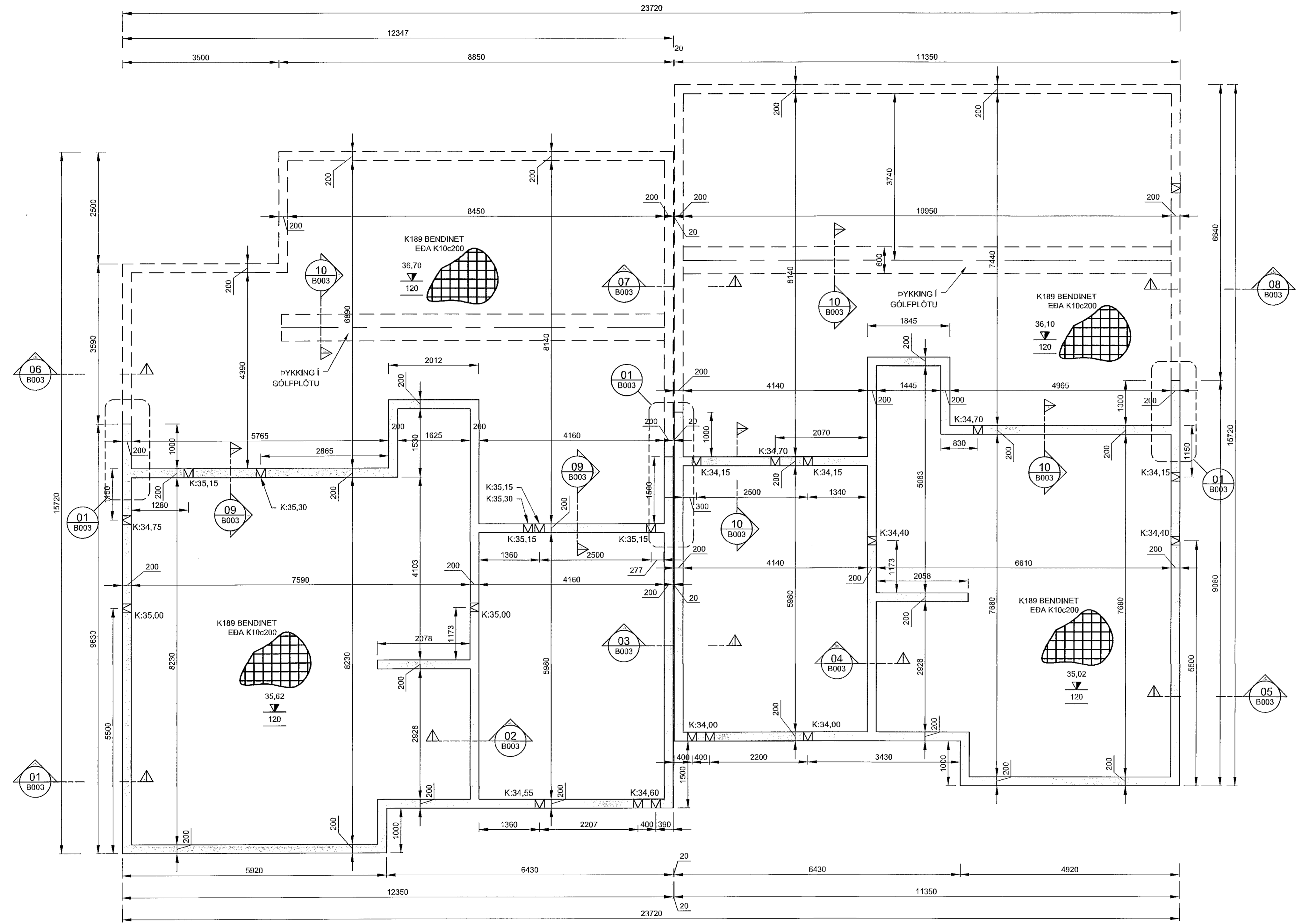
GRUNNMYND UNDIRSTÖÐUR - 1 1:50 (A1)
