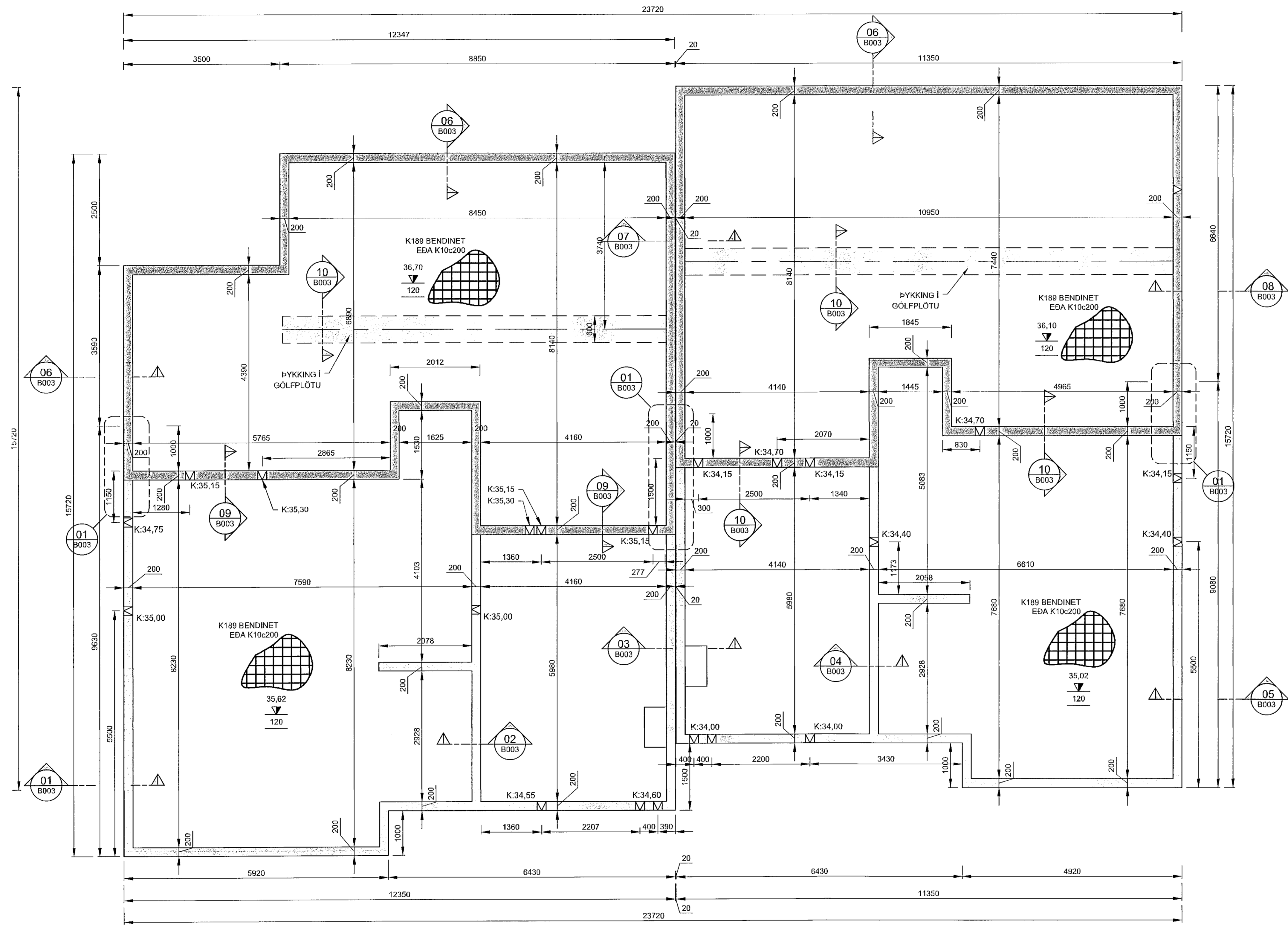
GRUNNMYND UNDIRSTÖÐUR - 2 1:50 (A1)
