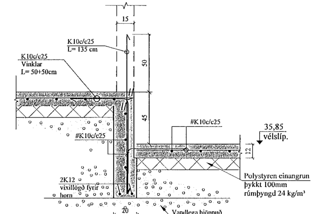
G2 SNIÐ. 1:20
