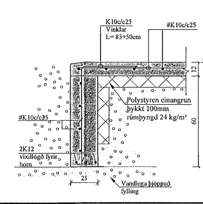
C2 SNIÐ. 1:20 Útveggur
