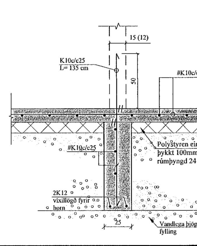
B2 SNIÐ. 1:20
