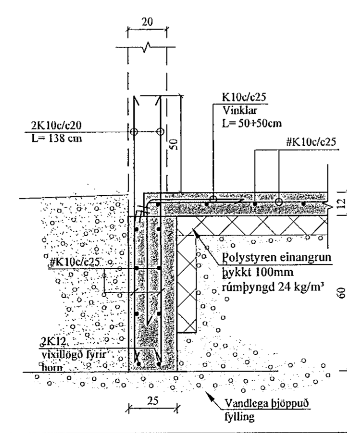
A2' SNIÐ. 1:20
