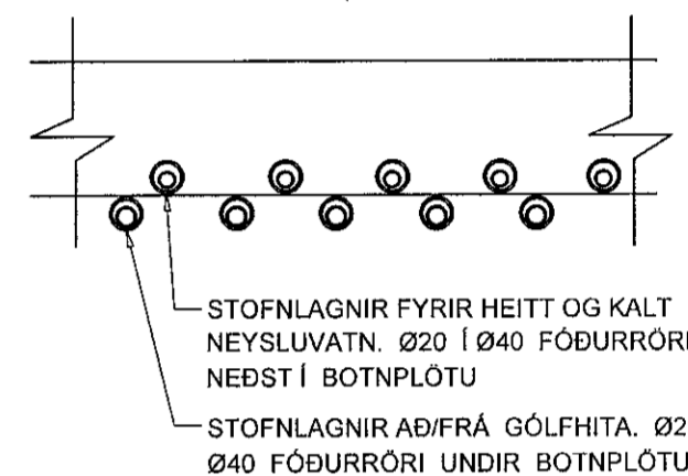
FÓÐURRÓR FYRIR GÓLFHITA OG NEYSLUVATN, KENNISNIÐ 1:10
