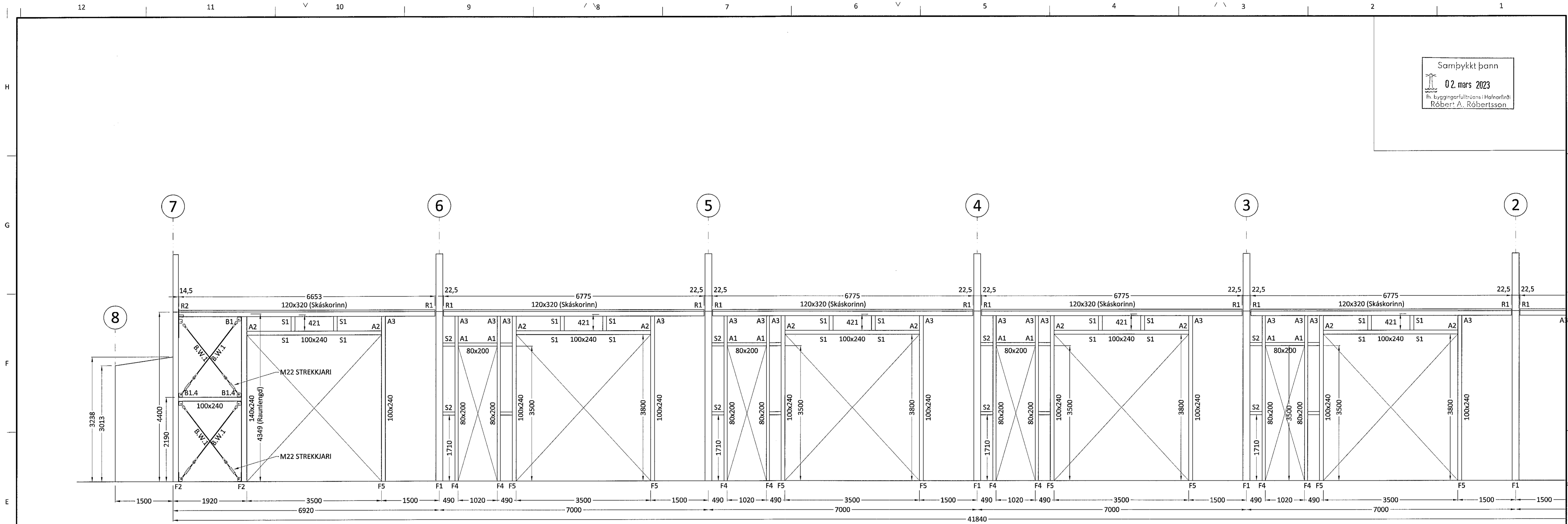
MODULE - B Mkv. 1:50
