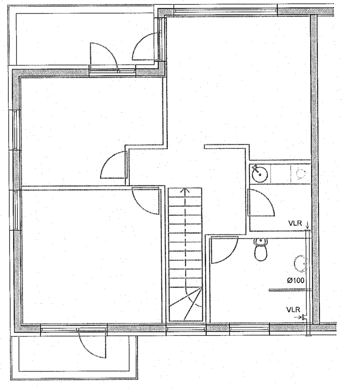
Grunnmynd 3. hæð, loftræsting 1:50
