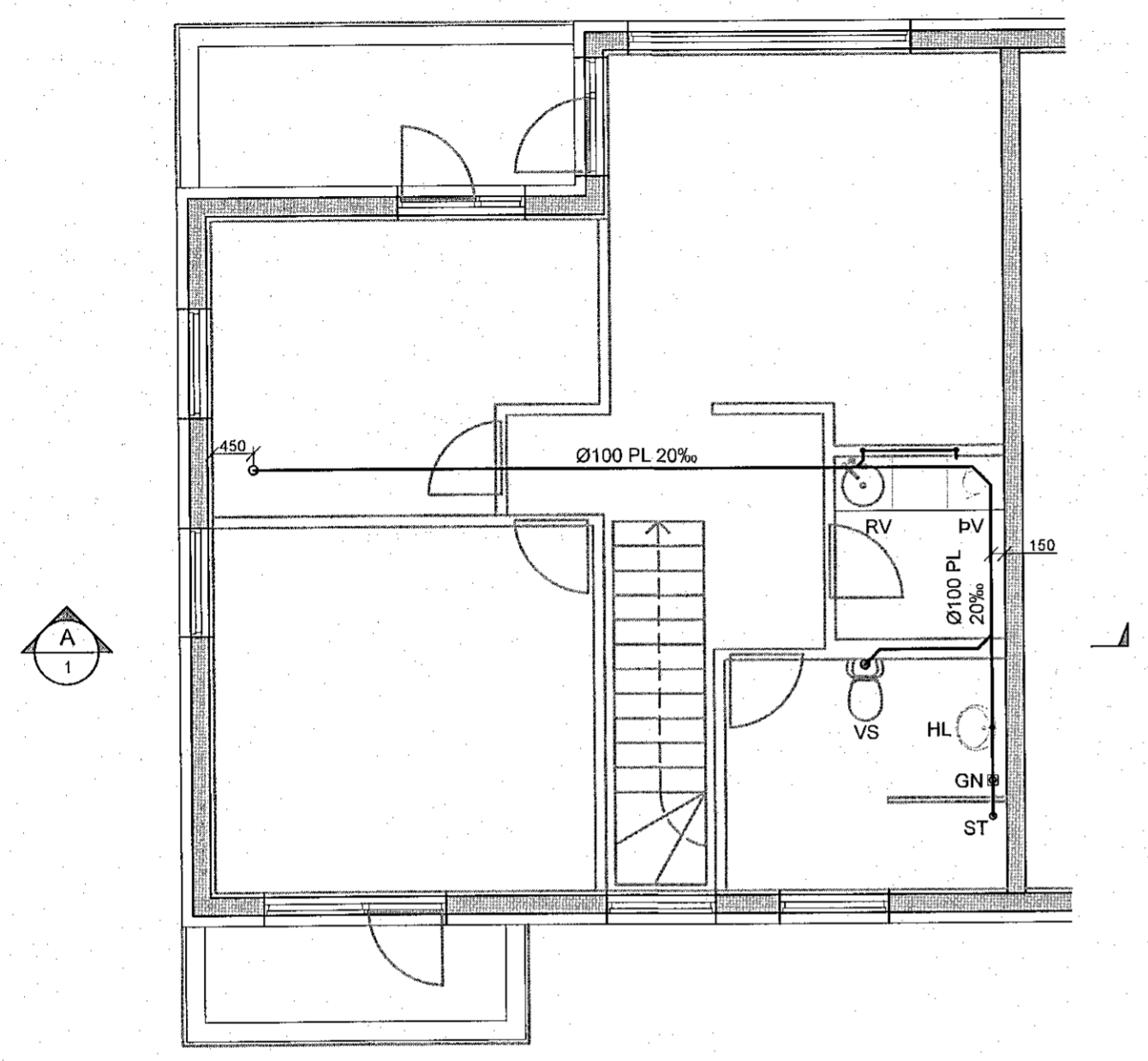
Grunnmynd 3. hæð, frárennsli 1:50
