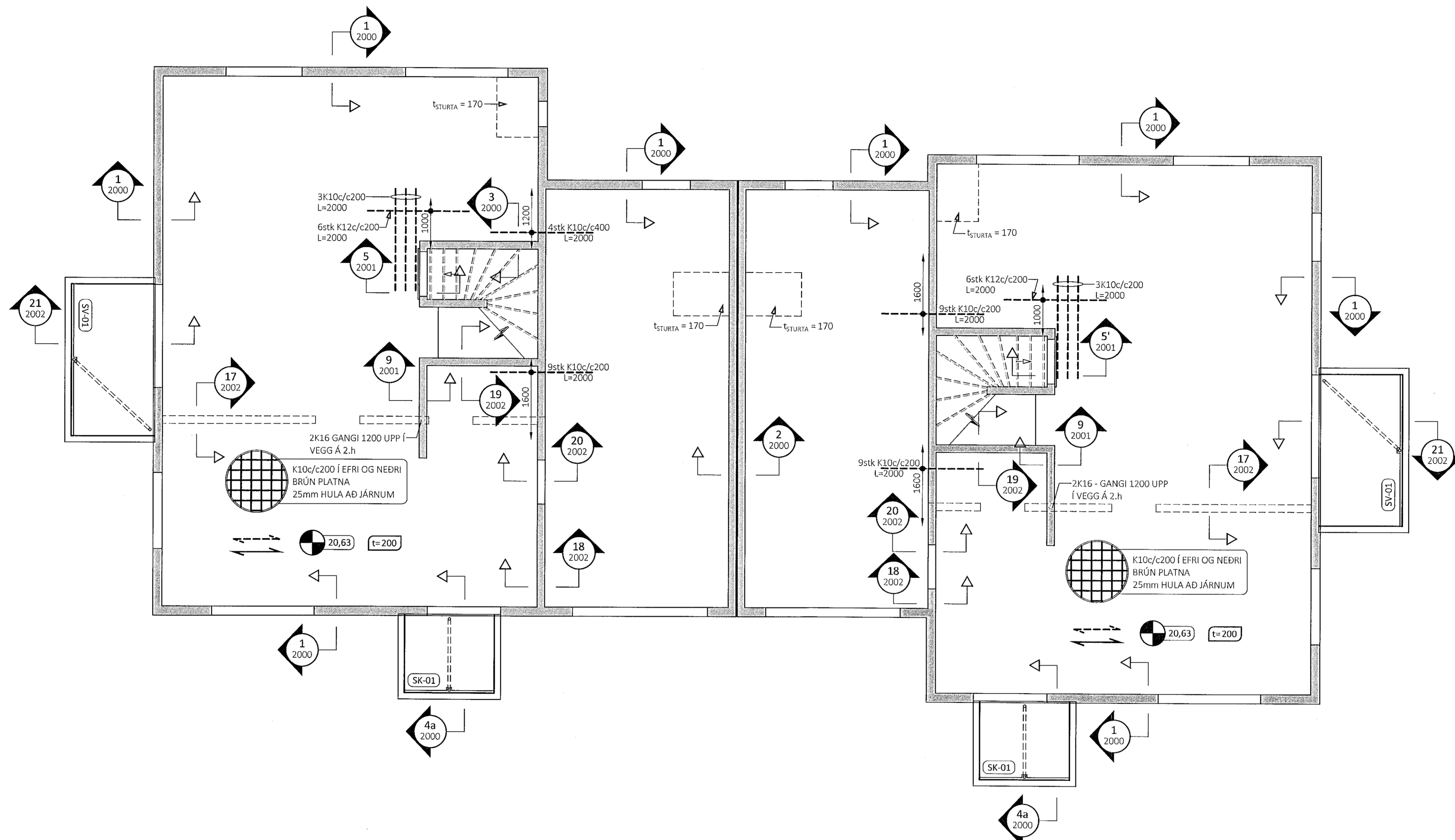
GRUNNMYND PLÖTU YFIR 1. HÆÐ - HÚS L TIL M - M1:50
