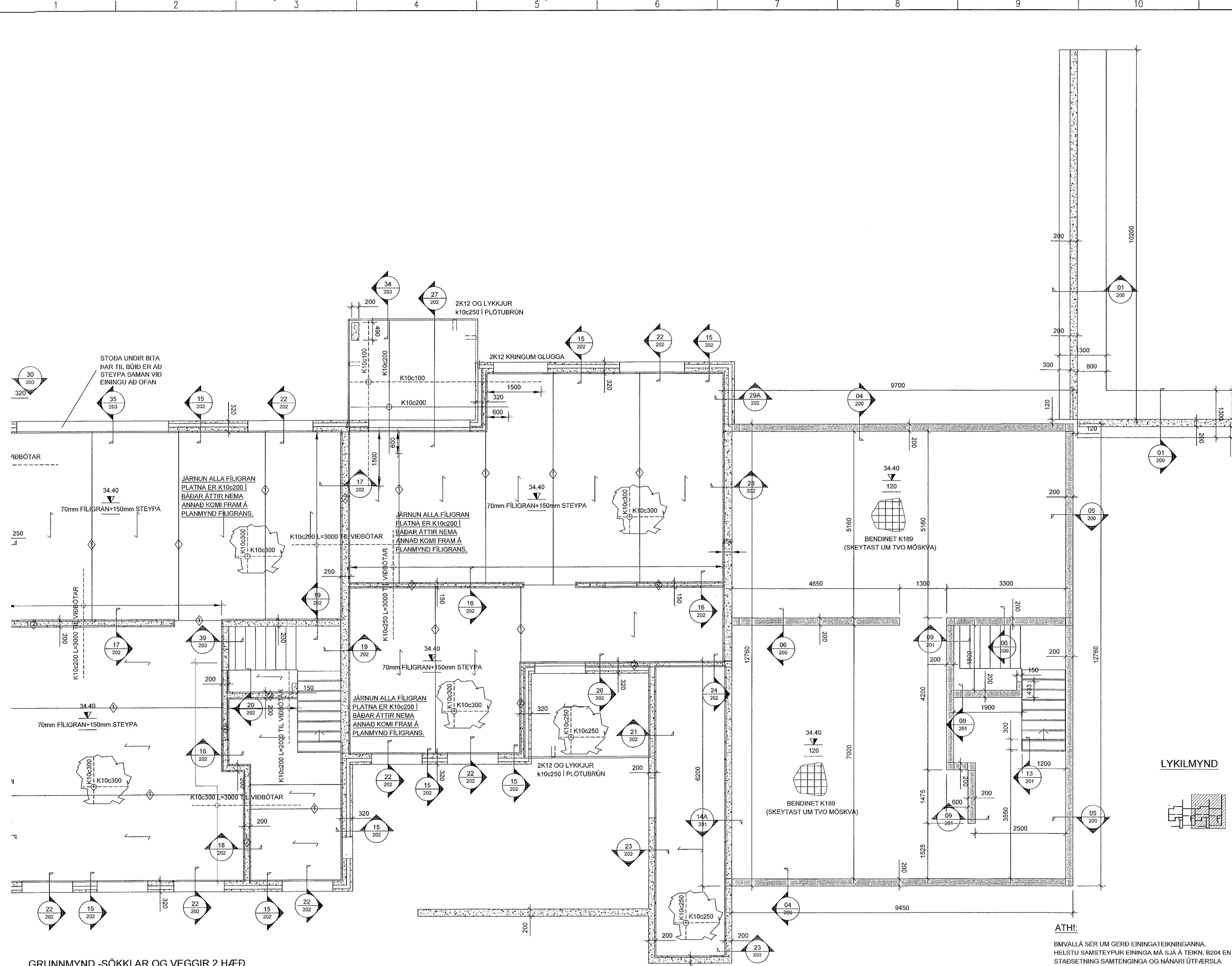
GRUNNMYND -SÖKKLAR OG VEGGIR 2.HÆÐ MKV. 3
