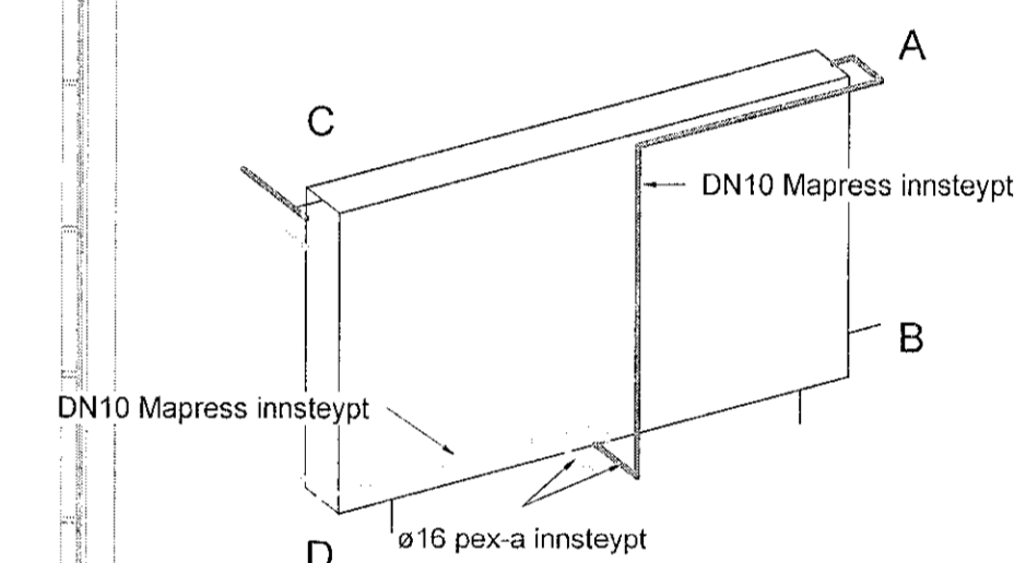
Dæmigerð tenging á ofni séð aftan frá
