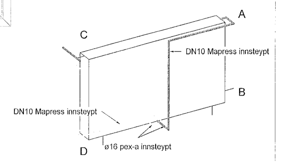
Dæmigerð tenging á ofni séð aftan frá
