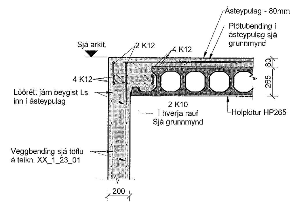
EA Snið EA 01.121.01 1 : 20
