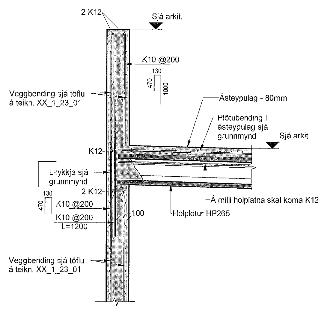
EH Snið EH 01.121.01 1 : 20
