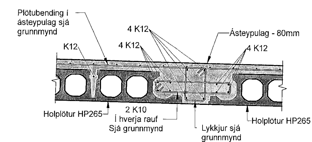
EG Snið EG 01.121.01 1 : 20
