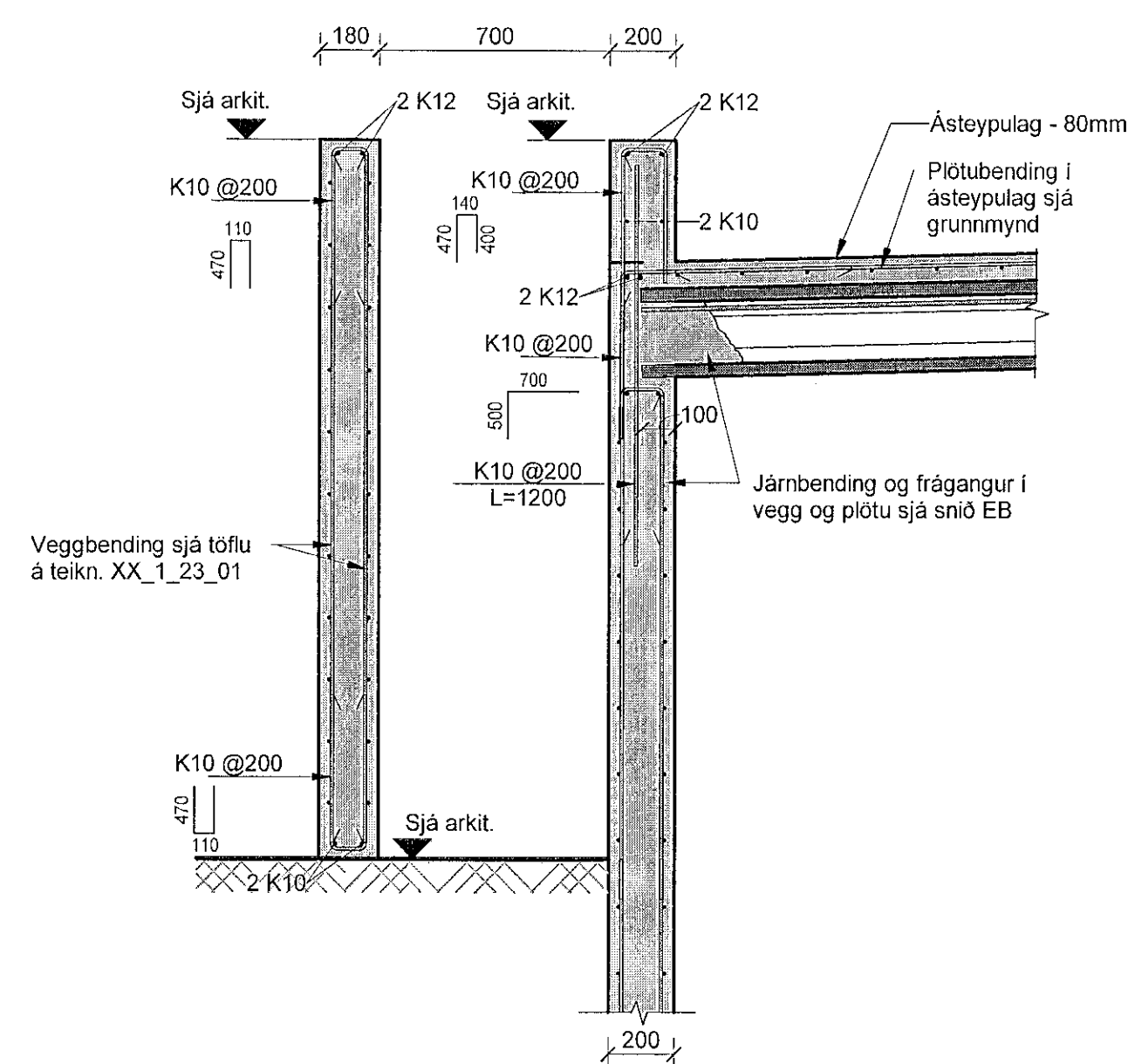
EF Snið EF 00.121.04 1 : 20
