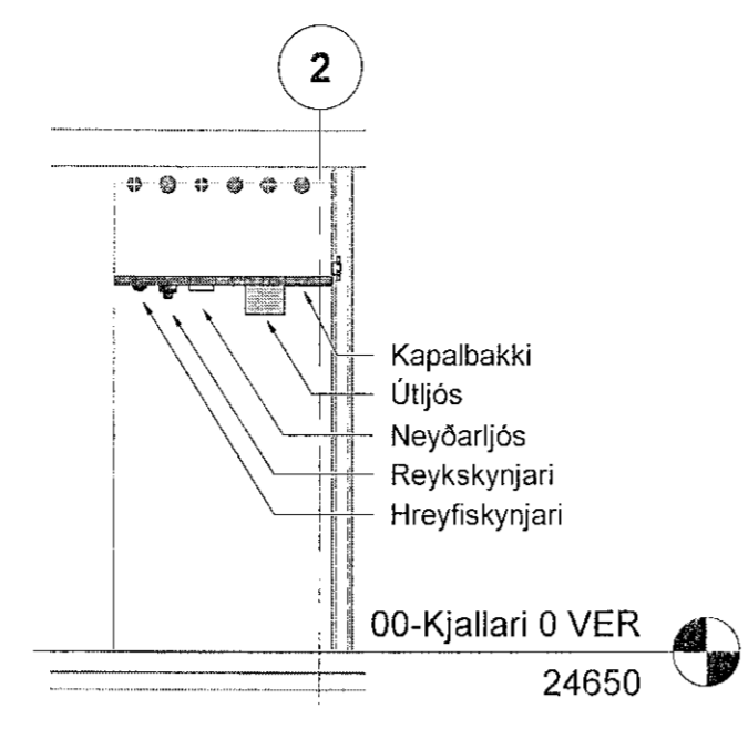
EC Snið EC 00_3_14_01 1 : 50
