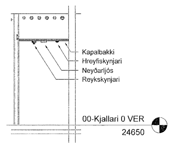
EE Snið EE 00_3_14_01 1 : 50
