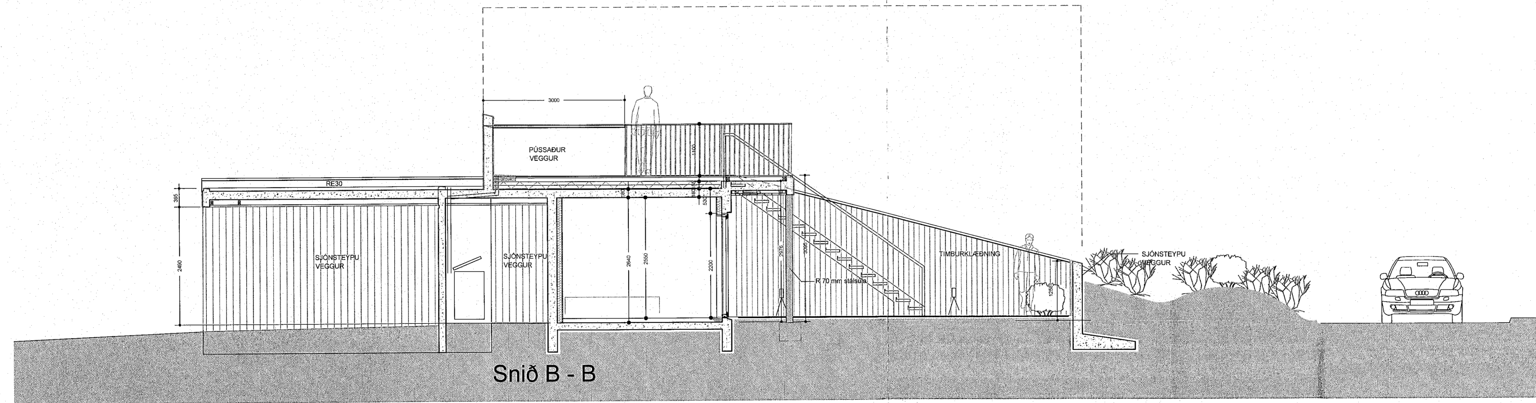
Snið B-B 1:50
