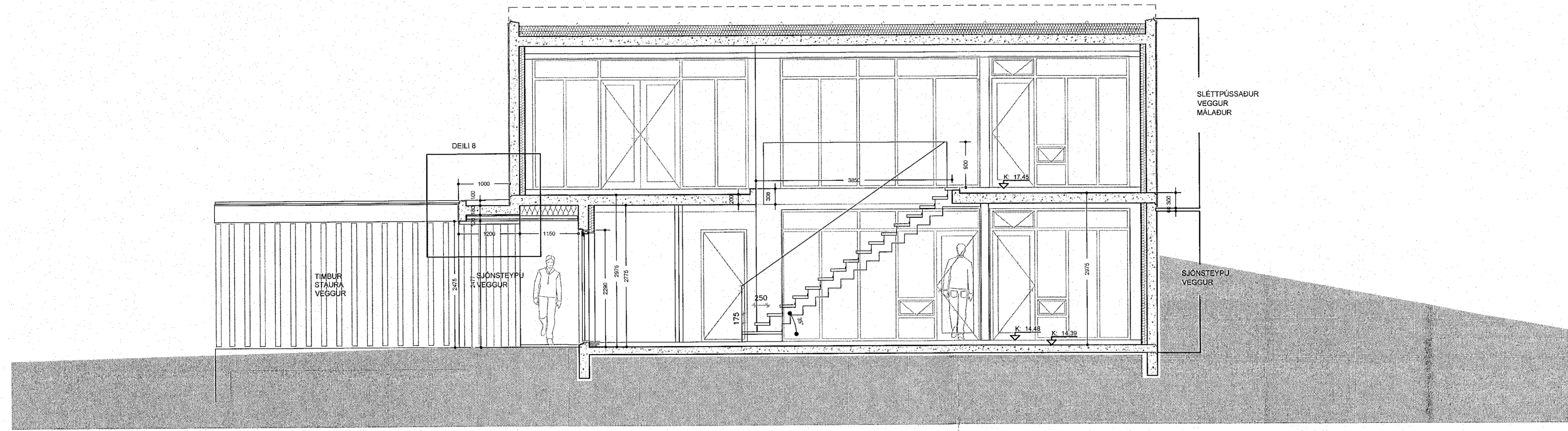
Snið A-A 1:50
