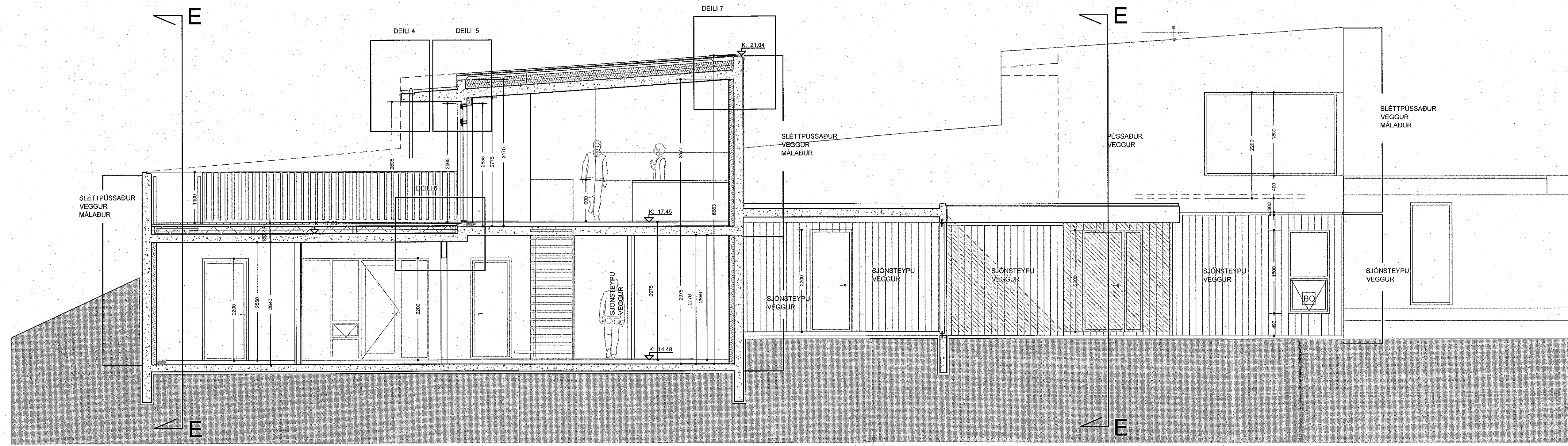
Snið C-C 1:50
