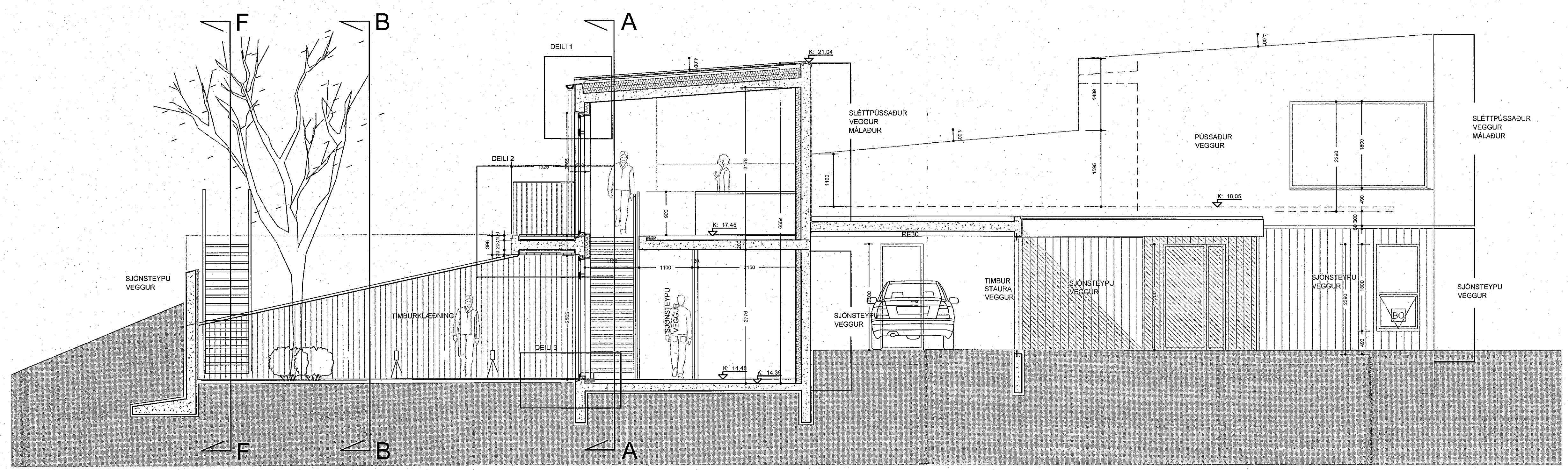
Snið D-D 1:50
