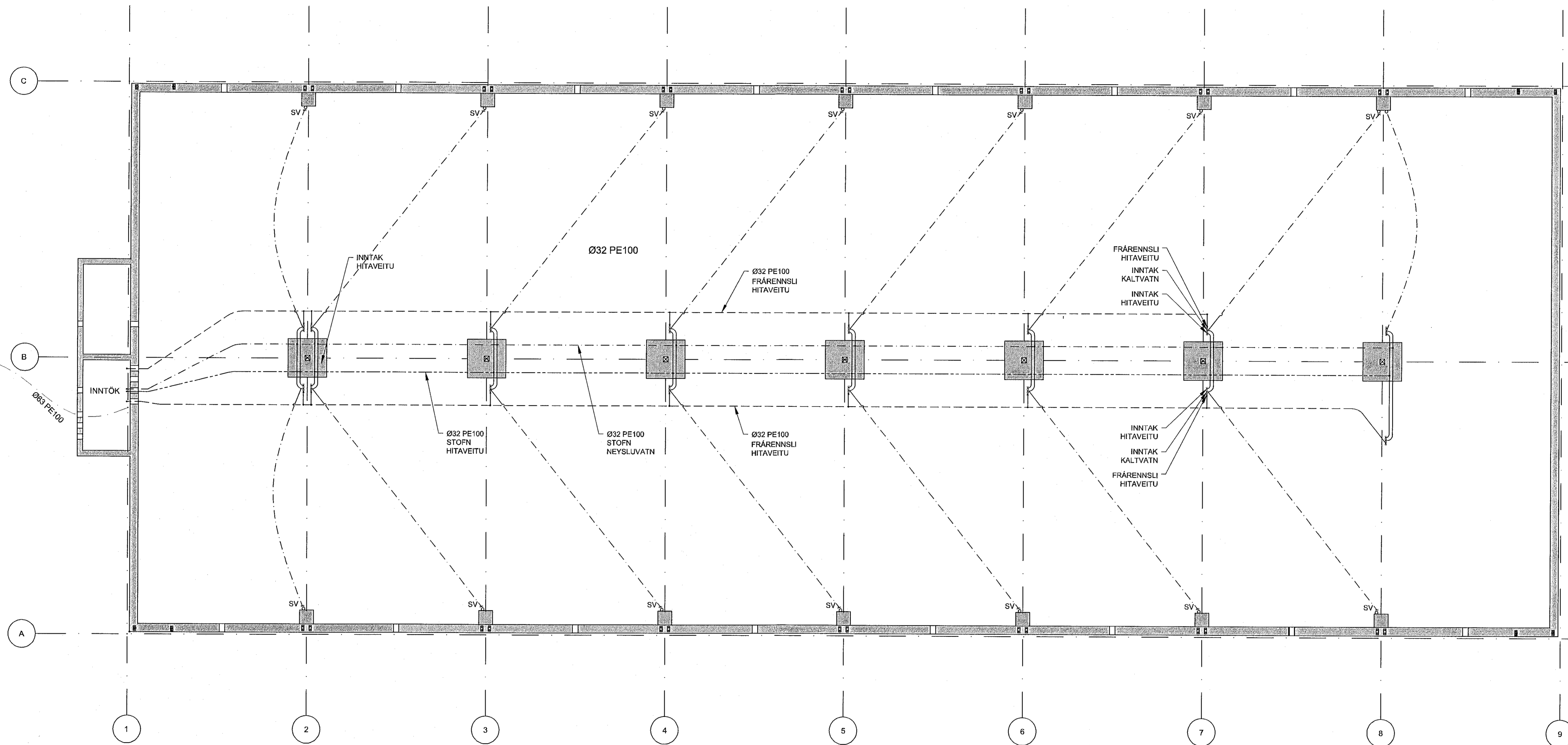
GRUNNMYND - NEYSLUVATNSLAGNIR 1:75 (A1)
