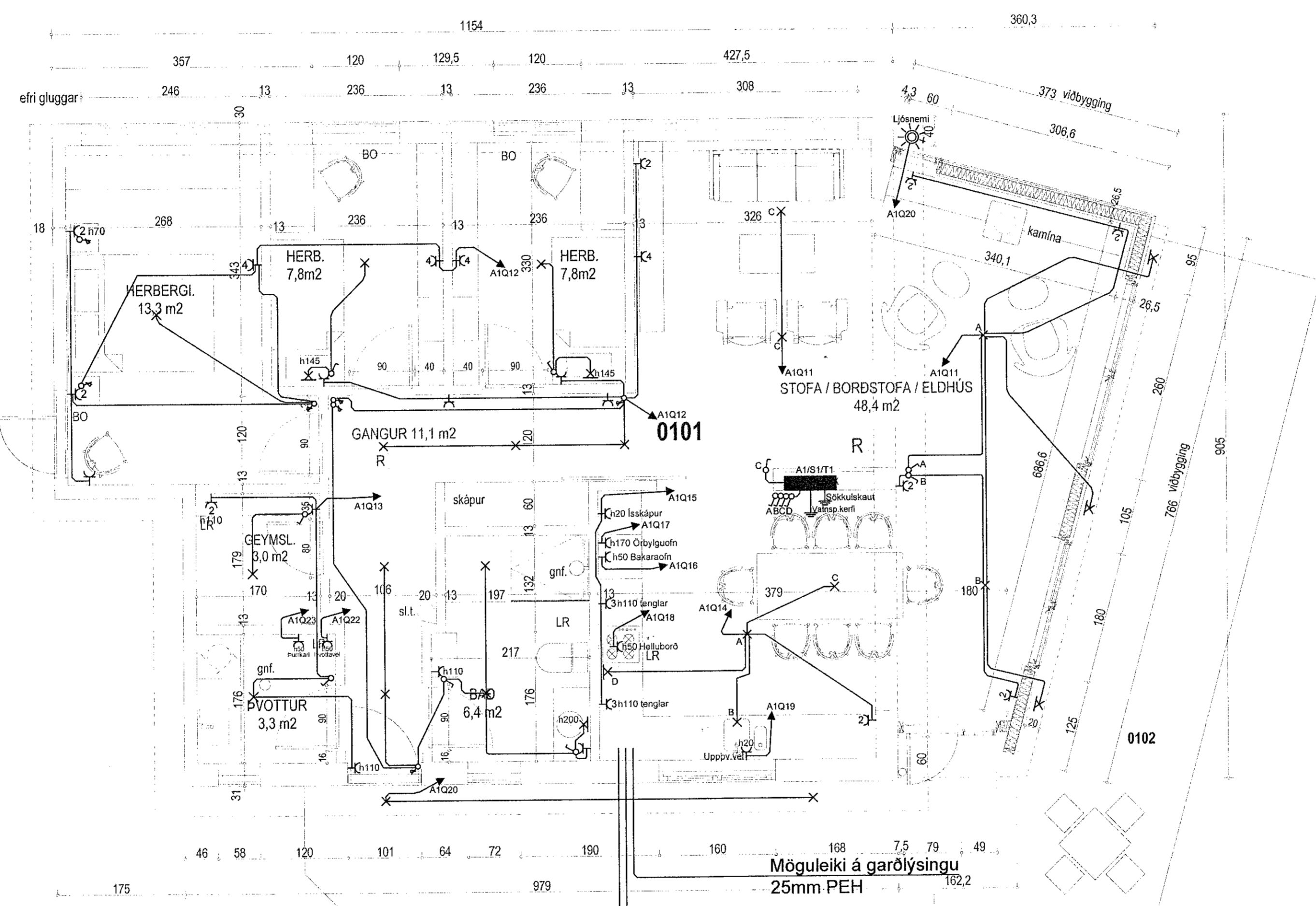
GRUNNMYND 1:50
