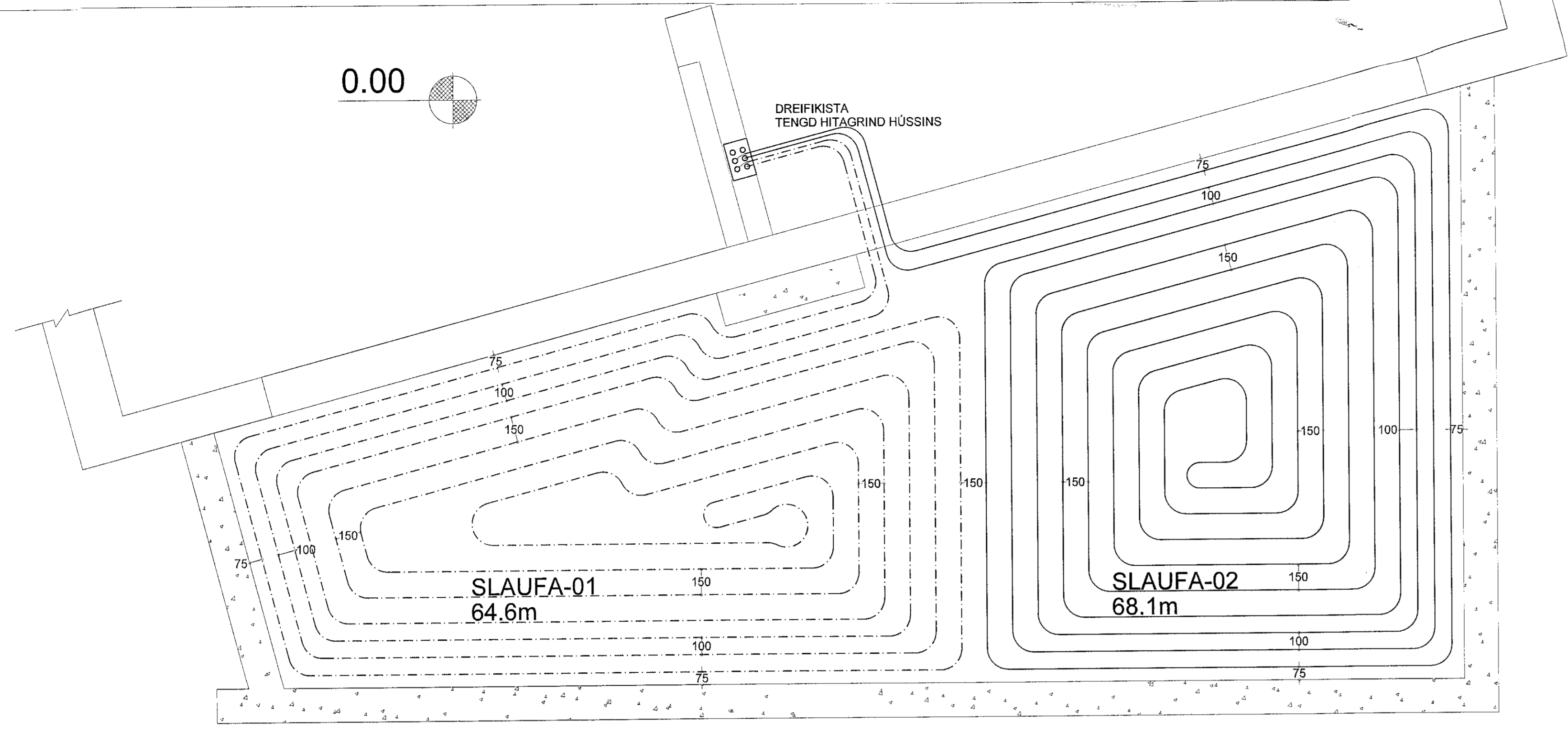
GÓLFHITALAGNIR mkv. 1:20
