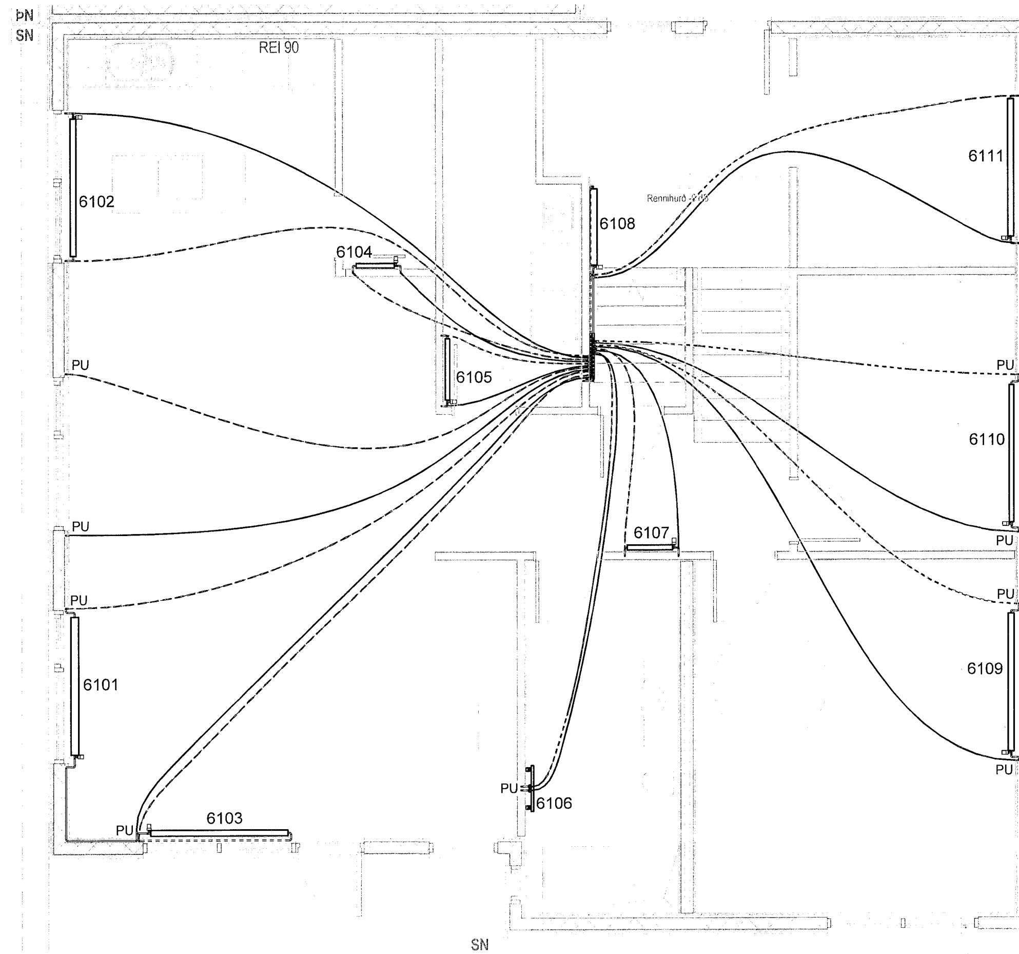
1. hæð - Grunnmynd 2 1 : 50
