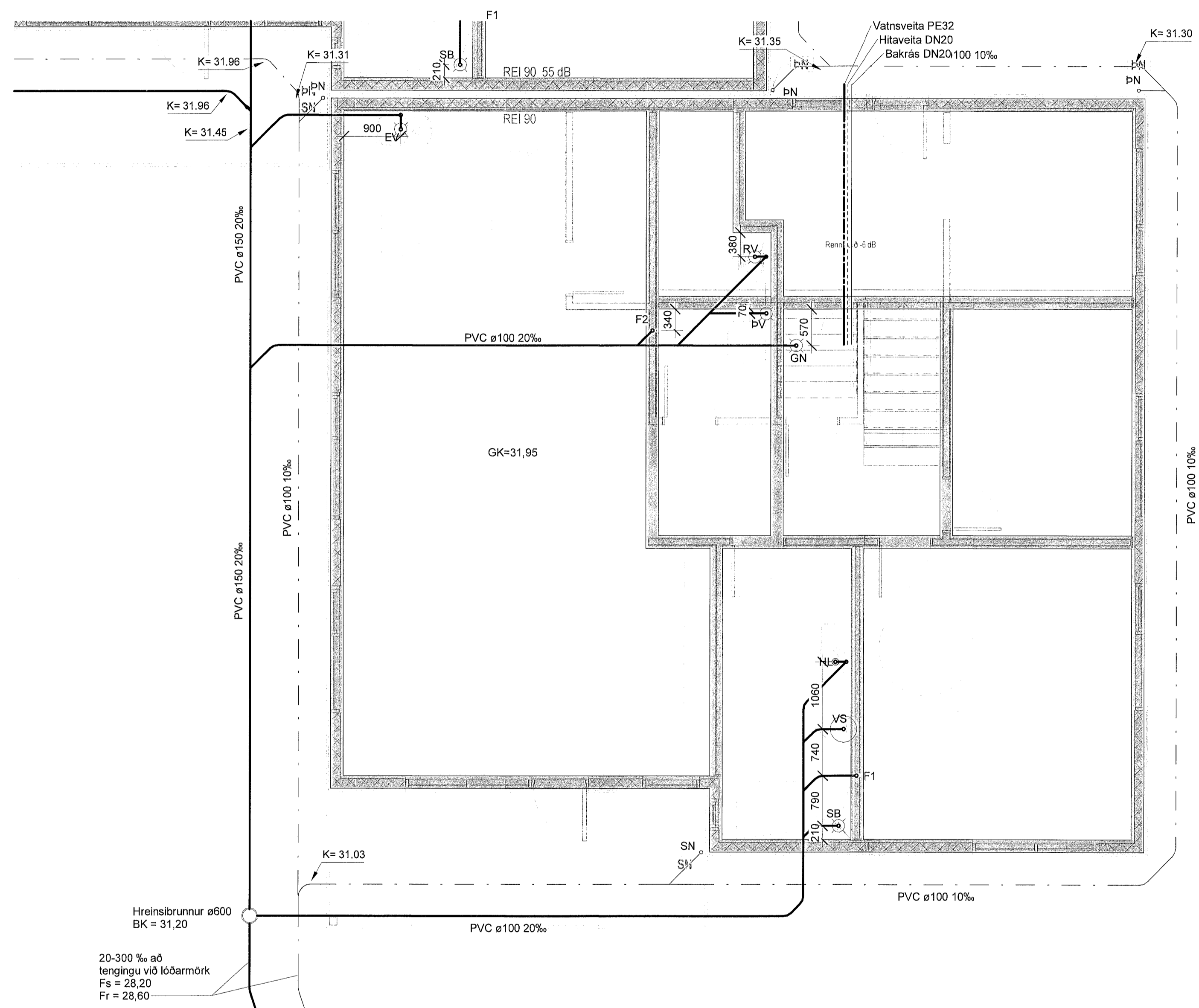
1. hæð - Grunnmynd 2 1 : 50
