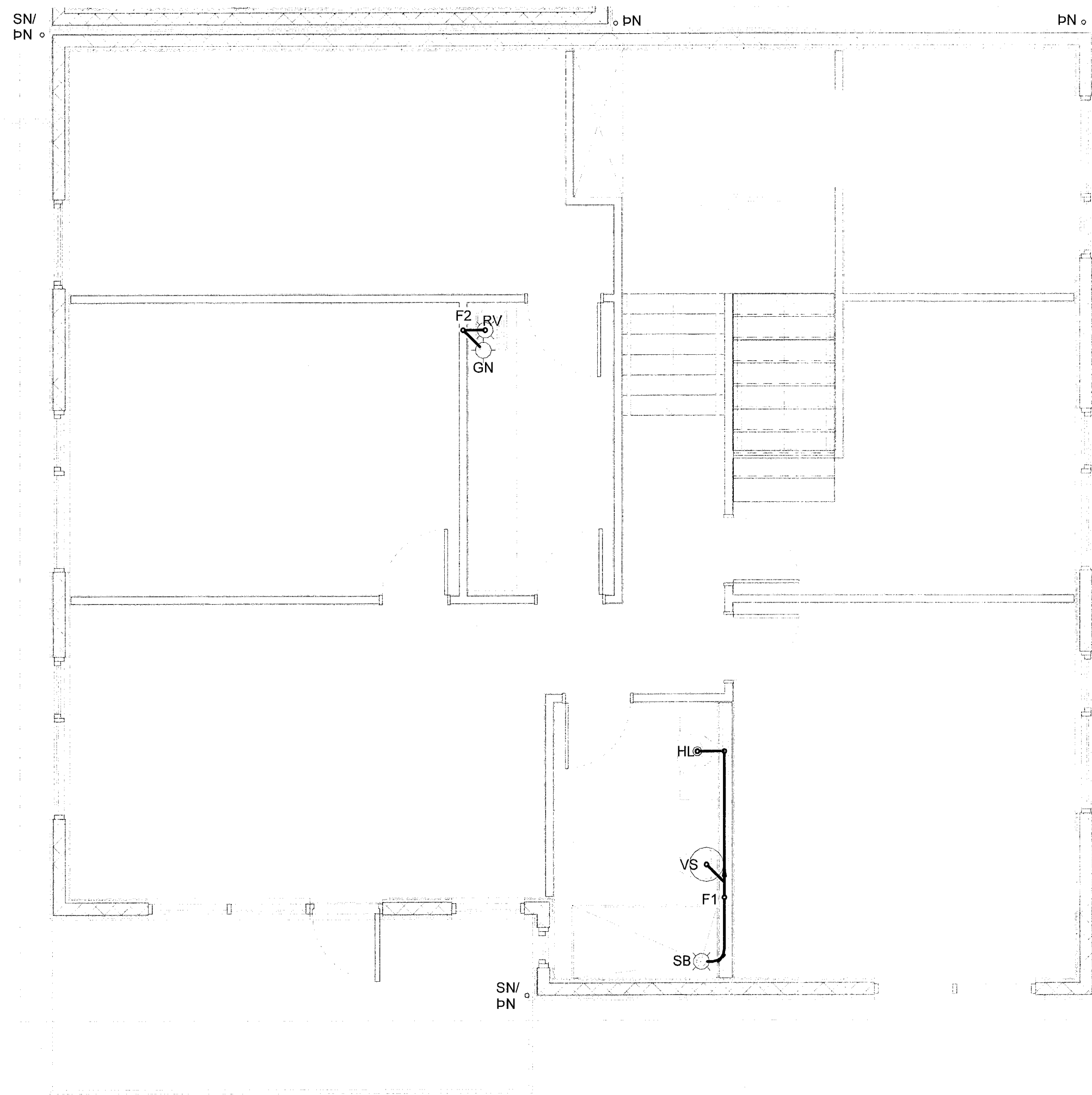
1 2. hæð - Grunnmynd 2 1 : 50
