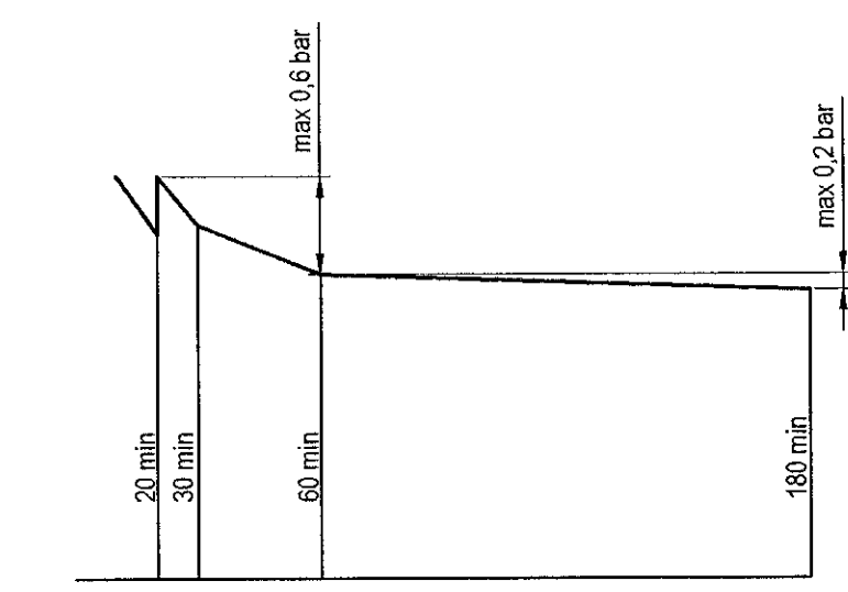
Þrýstiprófan á neysluvatslögnum línurit
