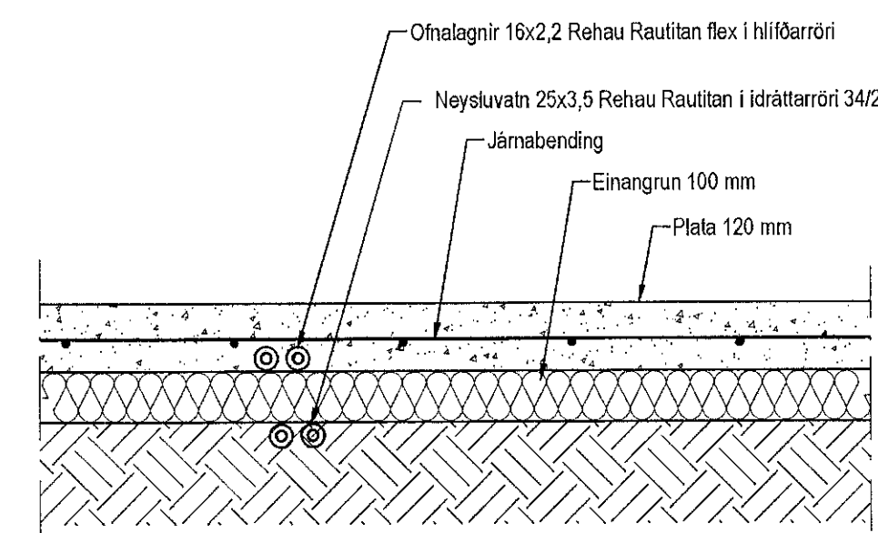
Hita- og vatnslagir, Snið í botnplötu, 1:10
