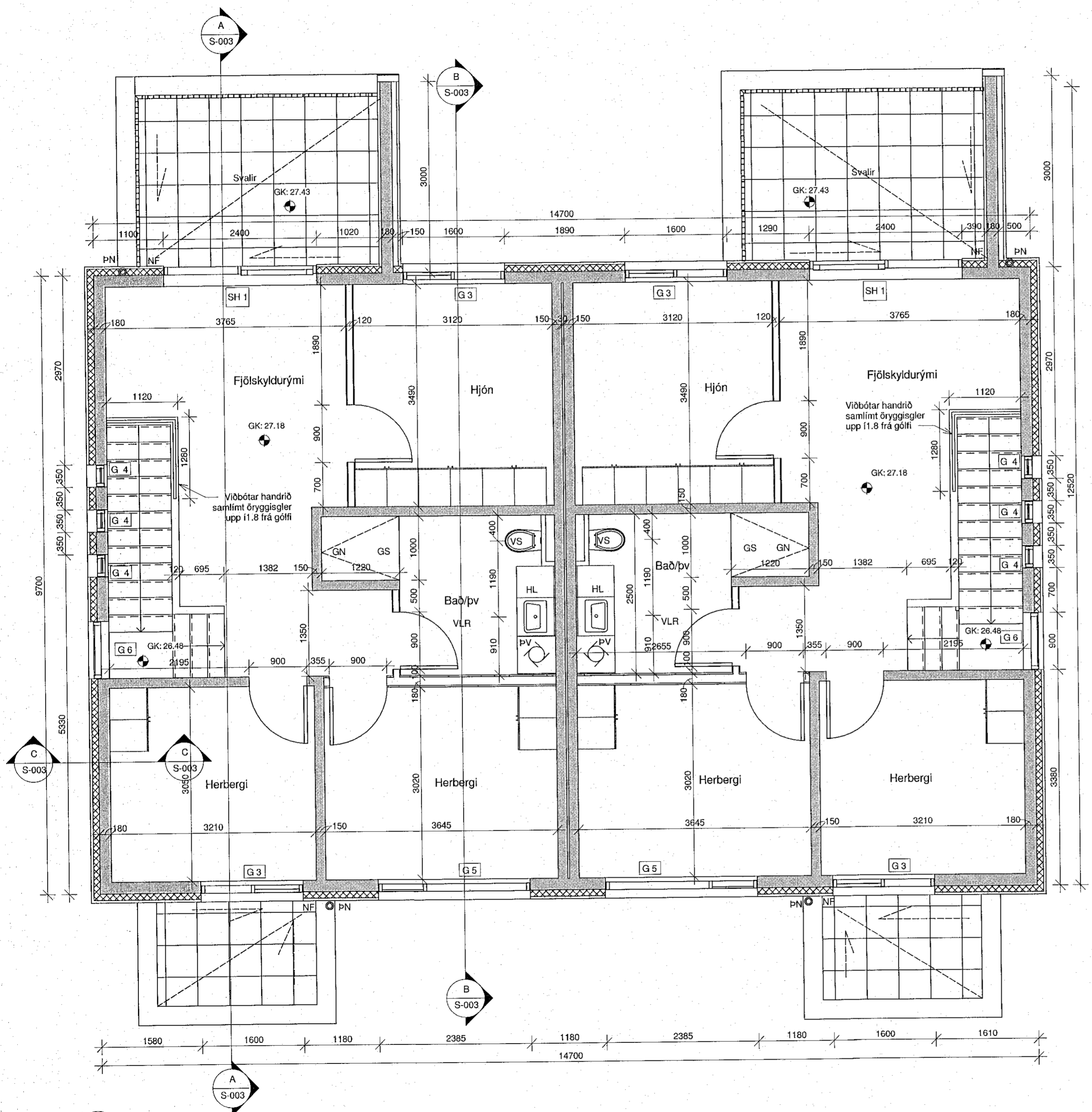
1 2.Hæð - 1/50 1:50
