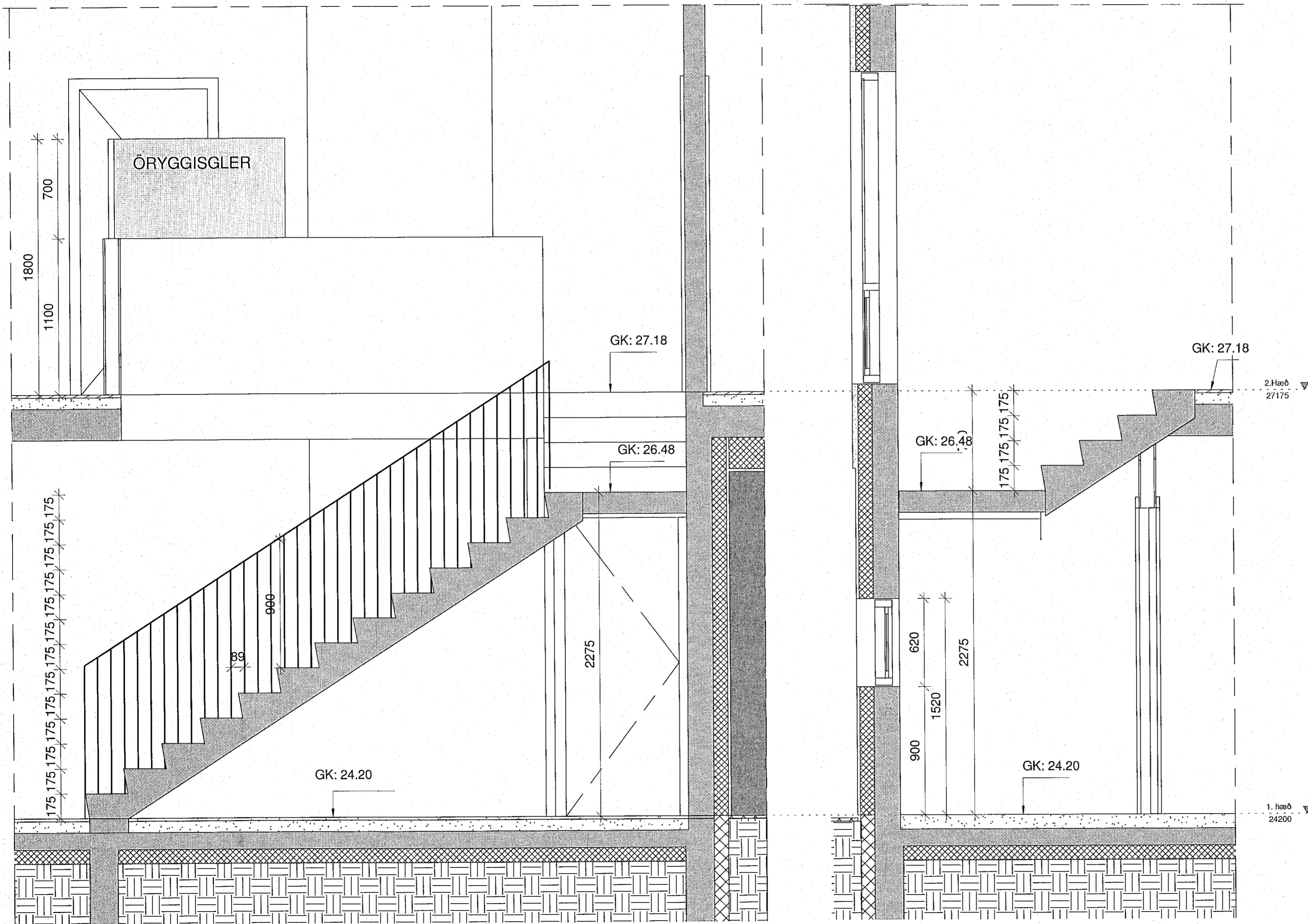
E Sneiðing E 1 : 20
