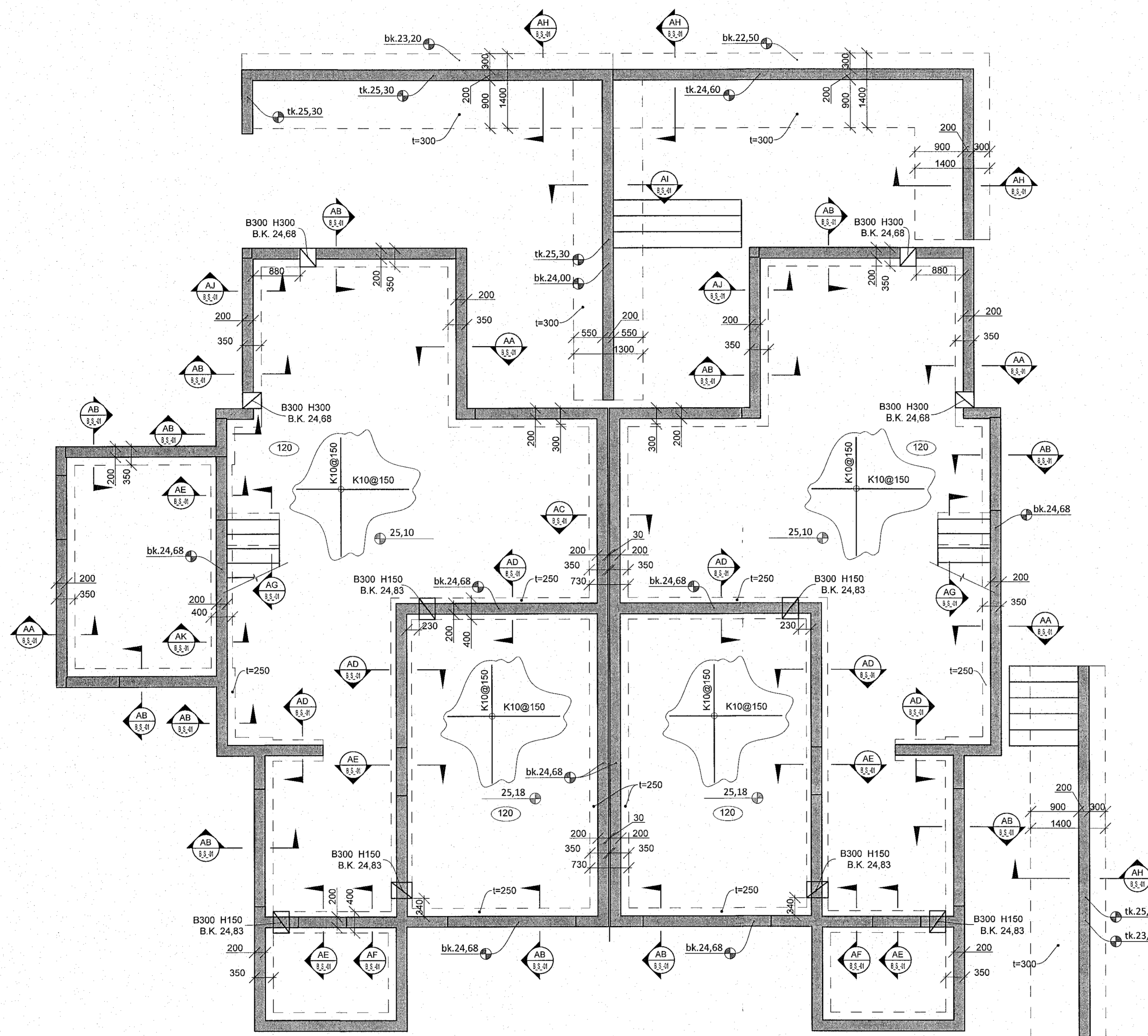
Grunnmynd - Sökklar M 1:50
