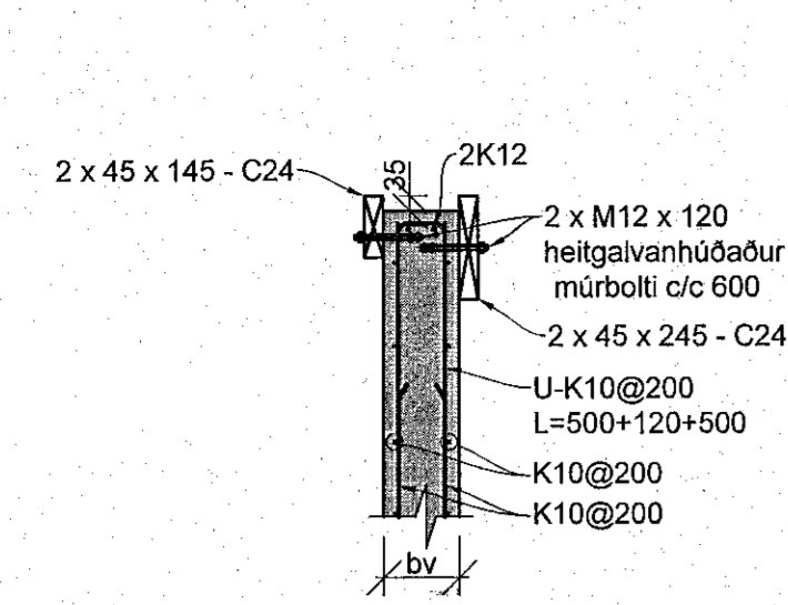
CA Pak við útvegg 1:20
