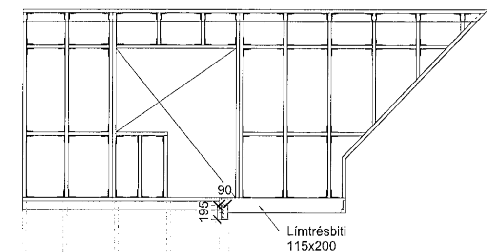
1 Grunnmynd - Milligólf og veggir 1.hæðar 1 : 50
