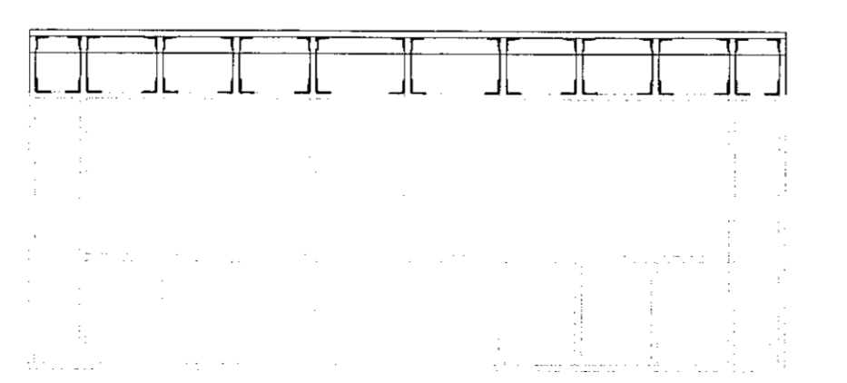
10 Útveggur norður 1 : 50
