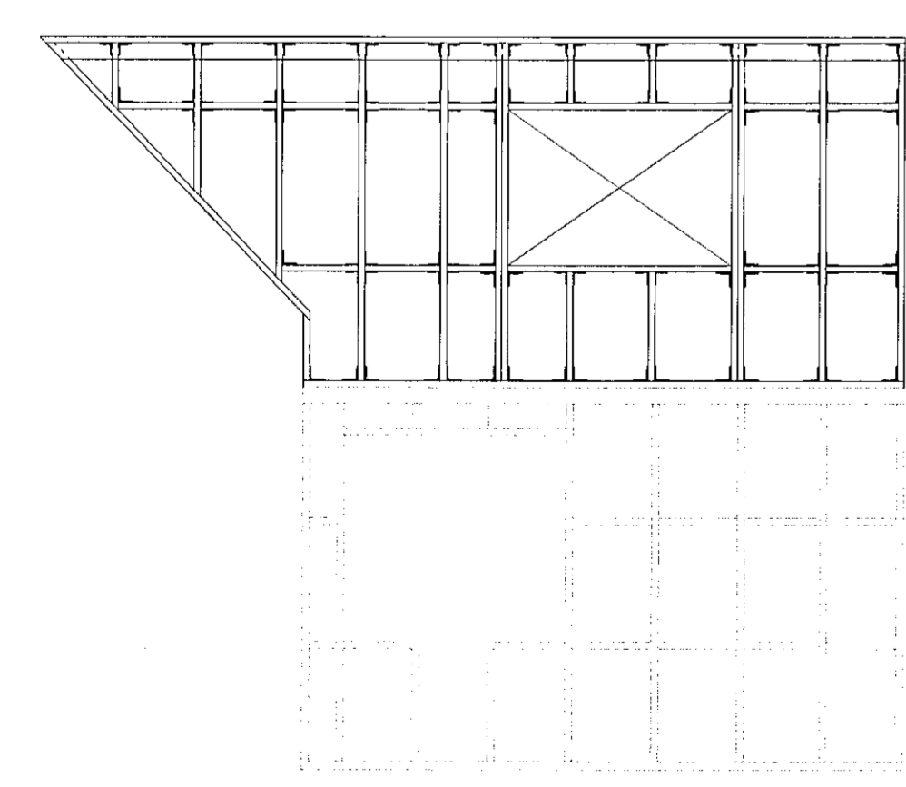
9 Útveggur vestur 1 : 50
