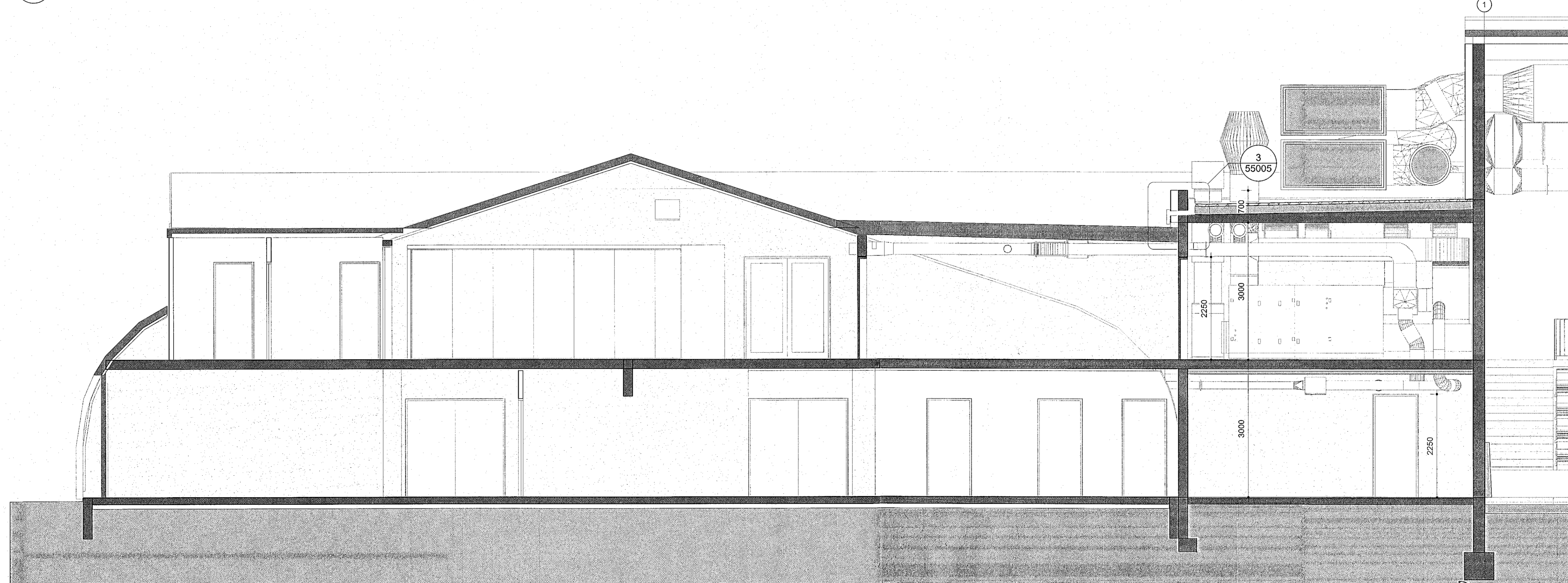
2 snið 42007 mkv: 1:50
