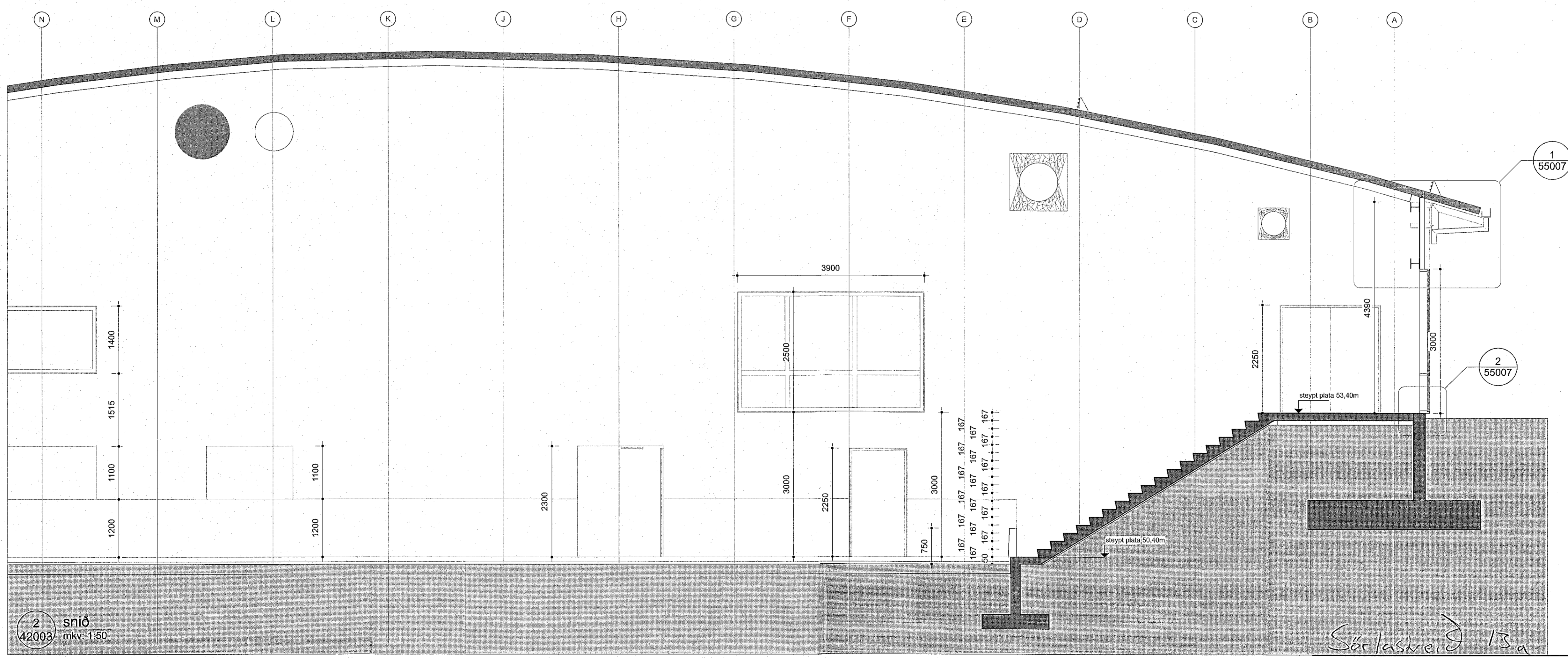
1 snið 42003 mkv. 1:50
