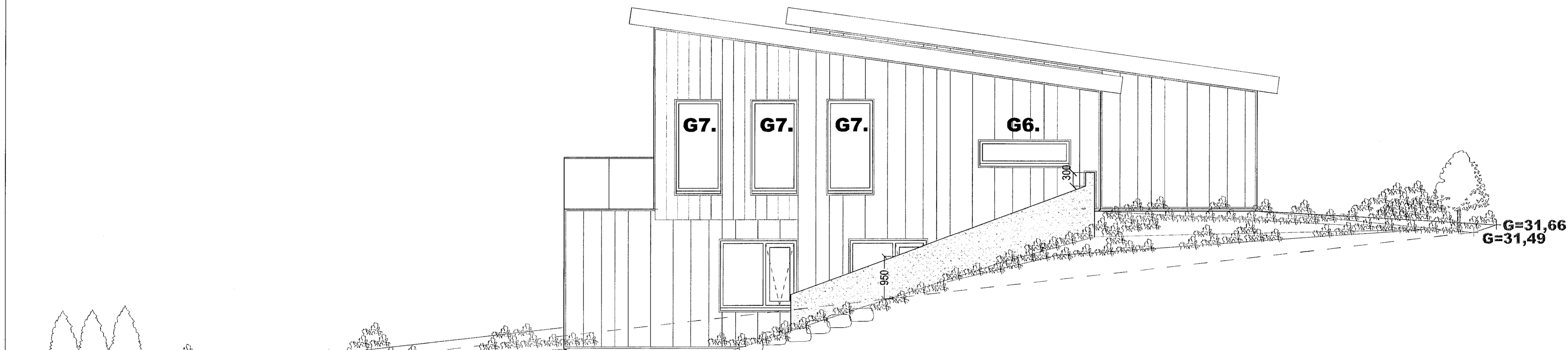
ÚTLIT AUSTUR MKV. 1:50.
