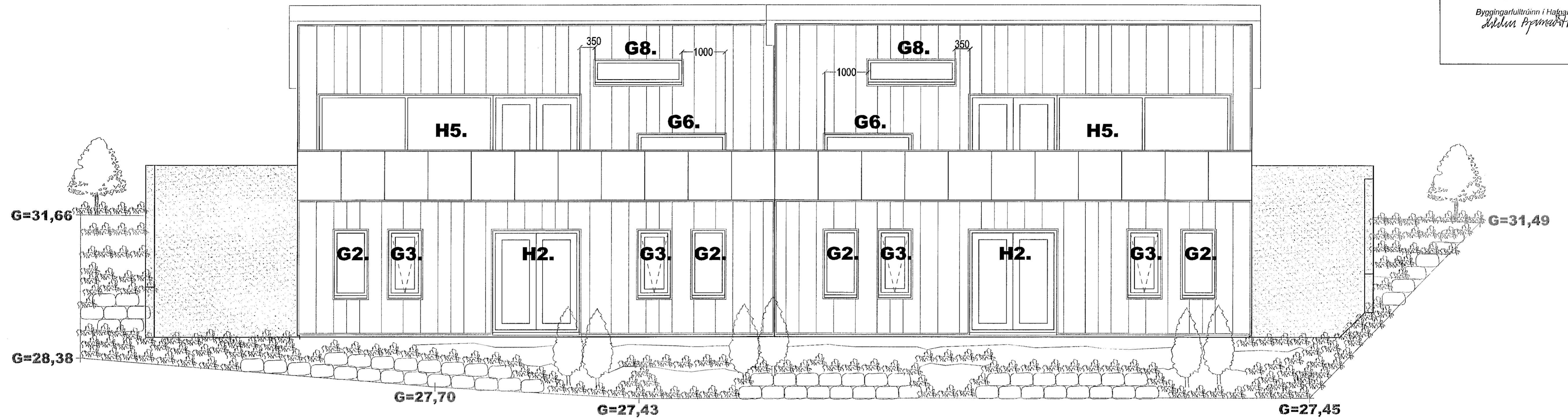
ÚTLIT SUÐUR MKV. 1:50.
