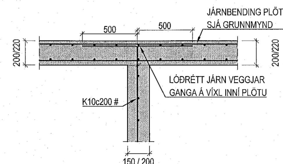
DÆMIGERT SNIÐ: TENING PLÖTU VID INNVEGGI ÞAR SEM EKKI ER VEGGAR FYRIR OFAN PLÖTU 1:20
