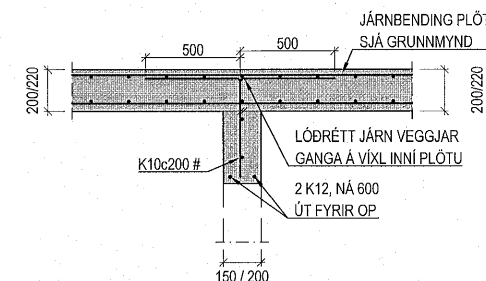
DÆMIGERT SNIÐ: TENING PLÖTU VID INNVEGGI, VID INNIHURÐIR, ÞAR SEM EKKI ER VEGGAR FYRIR OFAN PLÖTU 1:20
