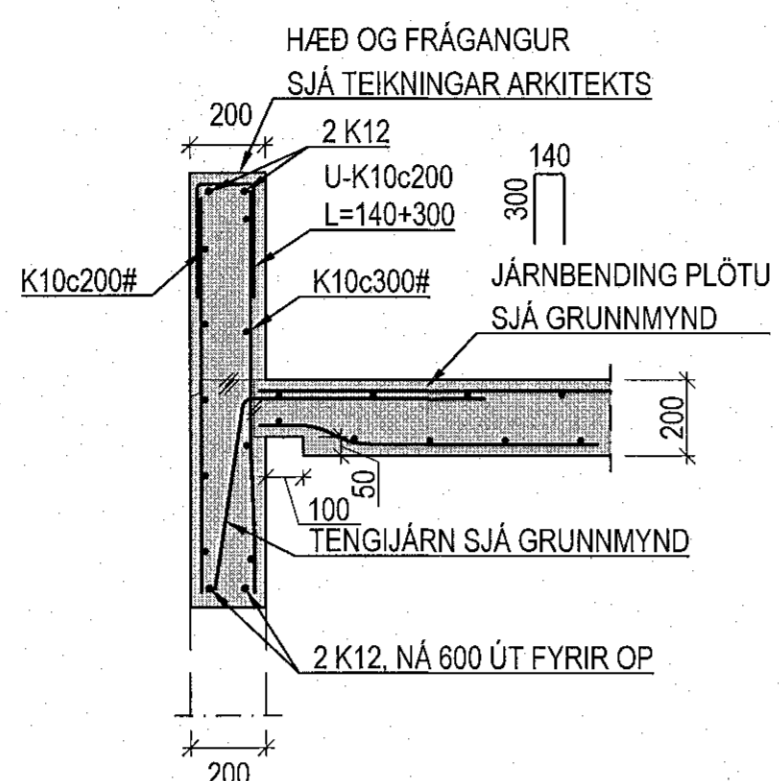
DÆMIGERT SNIÐ: TENING ÞAKPLÖTU VID ÚTVEGGI ÞAR SEM GLUGGAR ERU FYRIR NEDAN PLÖTU 1:20
