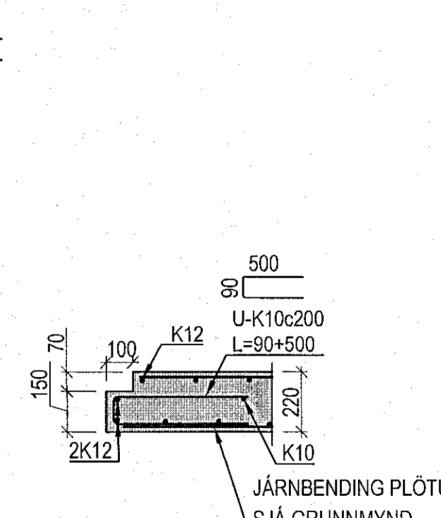
DÆMIGERT SNIÐ: ÚRTAK FYRIR LYFTUHURÐIR
