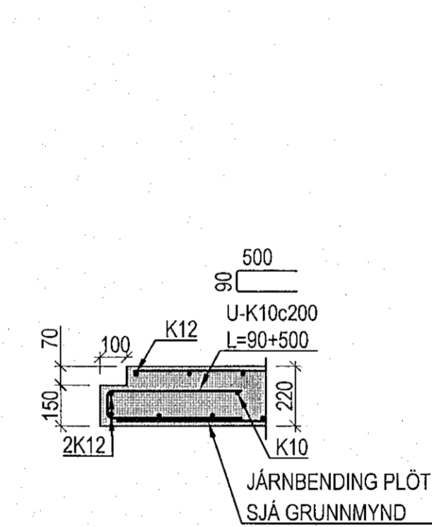
DÆMIGERT SNIÐ: ÚRTAK FYRIR LYFTUHURÐIR
