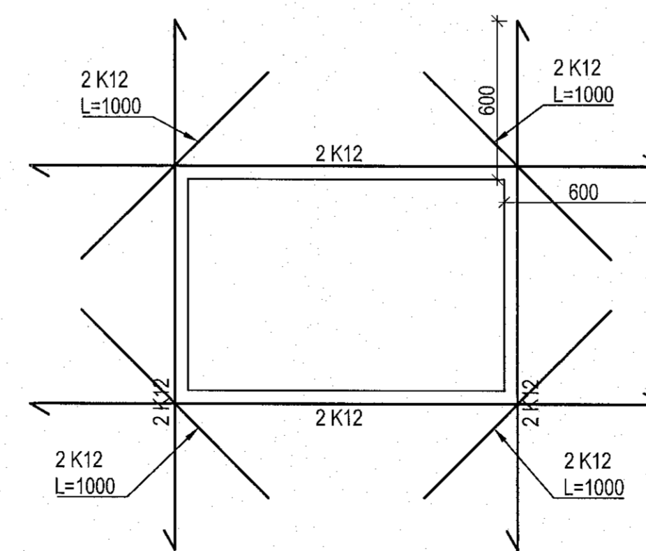
DÆMIGERT SNIÐ: JÄRNBENDING I KRINGUM GLUGGA OG HURÐIR 1:20
