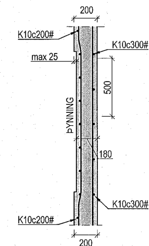
DÆMIGERT SNIÐ: JÄRNBENDING VID PYNNINGAR 1:20
