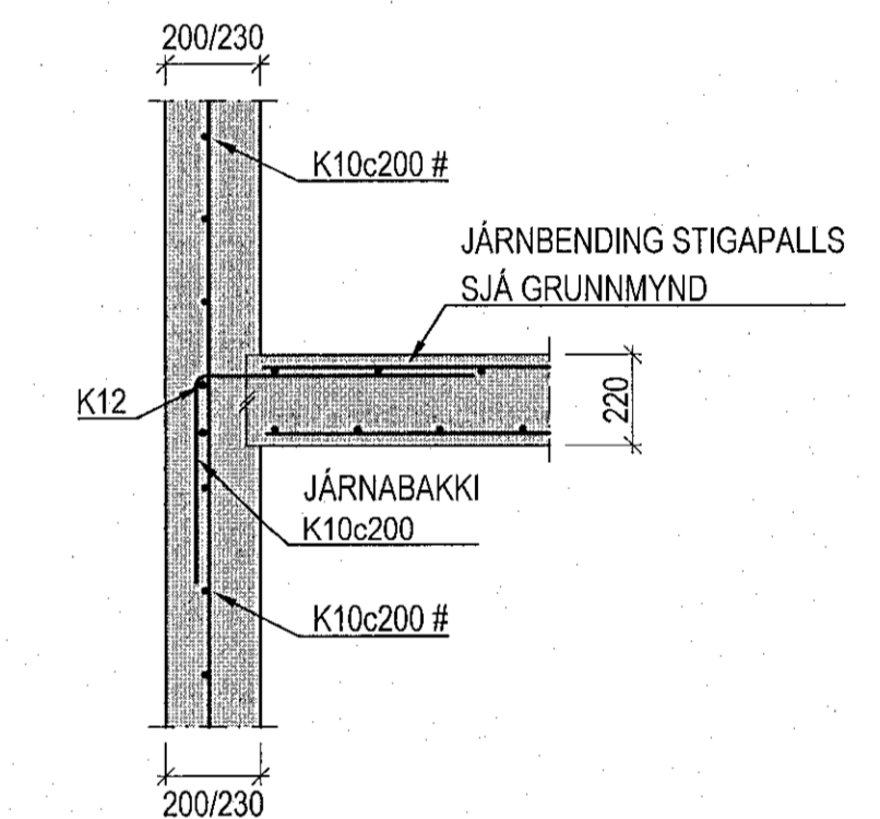
DÆMIGERT SNIÐ: TENING STIGAPALLS VID INNVEGGI
