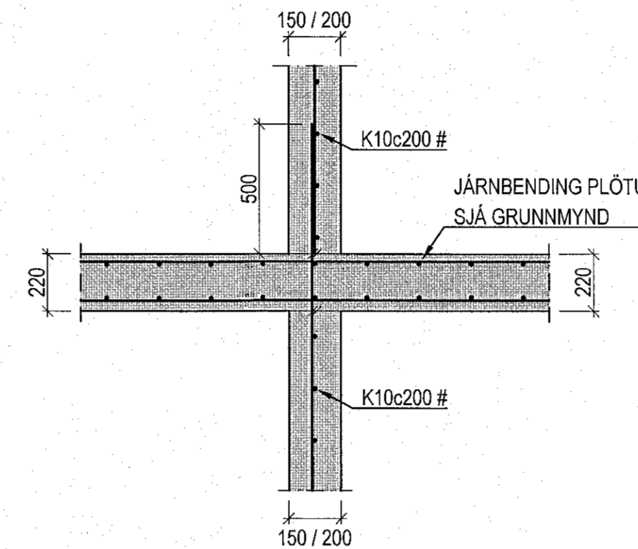
DÆMIGERT SNIÐ: TENING PLÖTU VID INNVEGGI 1:20
