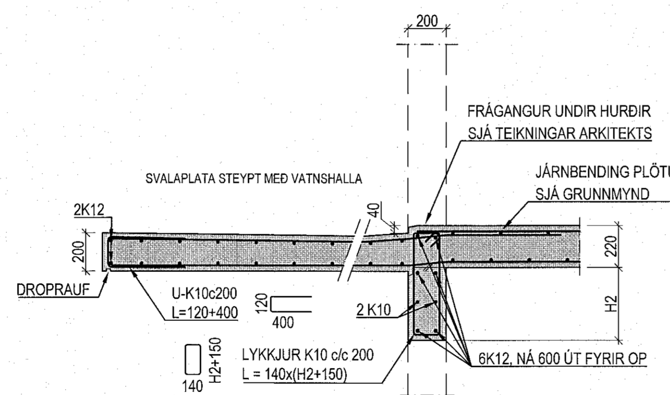
DÆMIGERT SNIÐ: TENING MILLIPLÖTU VID ÚTVEGGI VID SVALAHURÐIR / GÓLFSÍÐA GLUGGA 1:20
