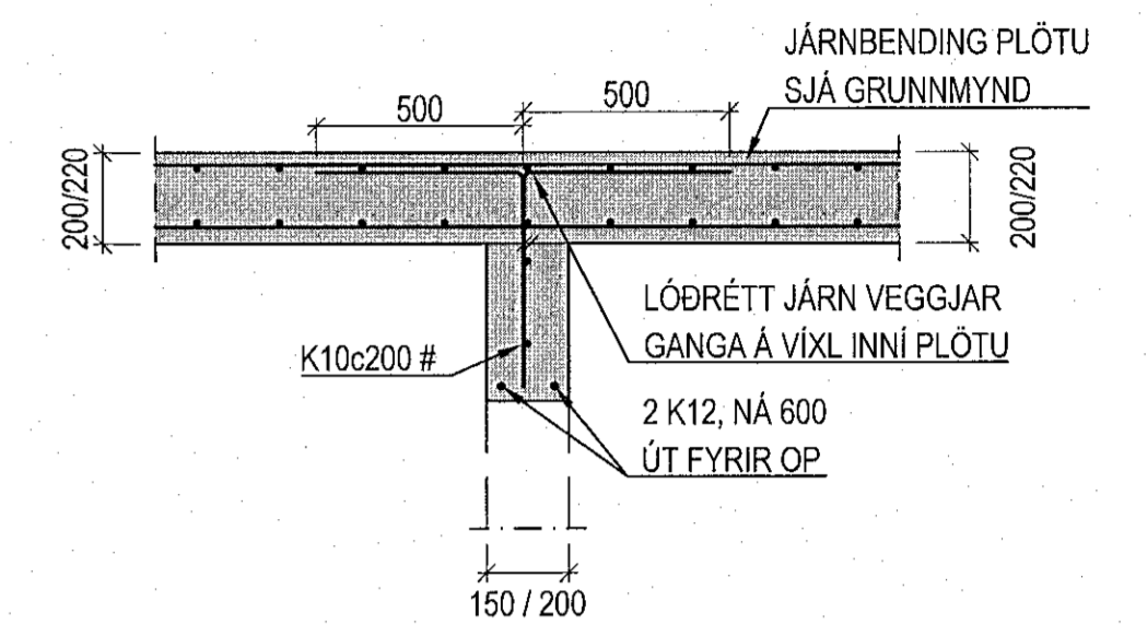
DÆMIGERT SNIÐ: TENING PLÖTU VID INNVEGGI, VID INNHURÐIR, ÞAR SEM EKKI ER VEGGUR FYRIR OFAN PLÖTU 1:20
