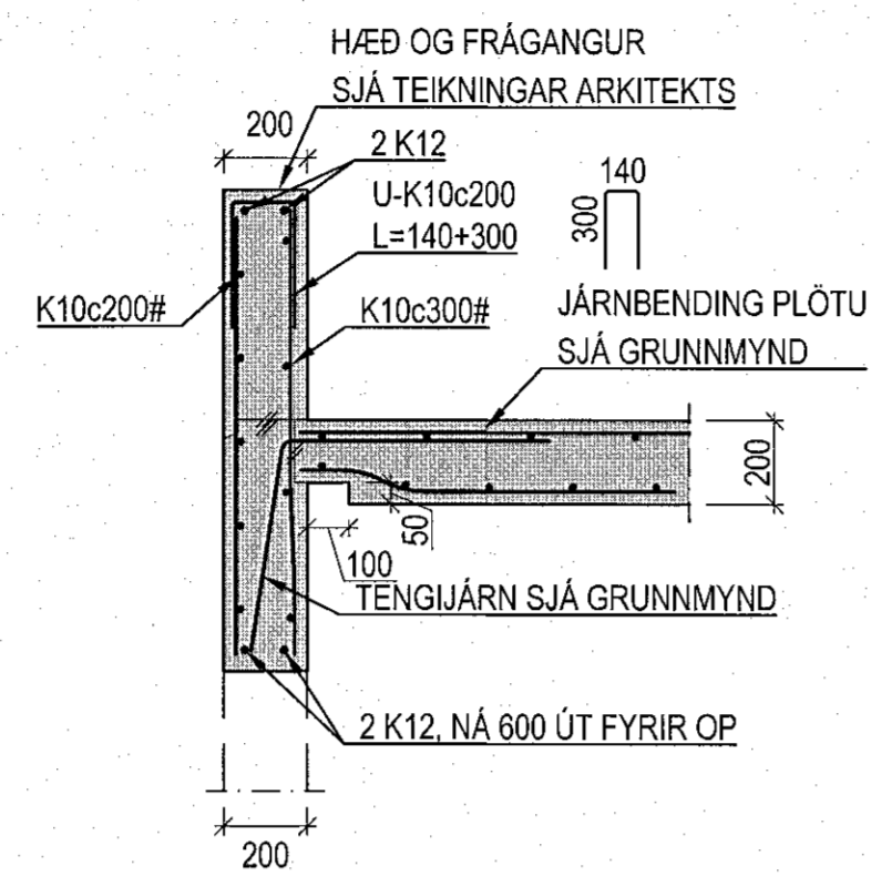
DÆMIGERT SNIÐ: TENING PAKPLÖTU VID ÚTVEGGI ÞAR SEM GLUGGAR ERU FYRIR NEDAN PLÖTU 1:20
