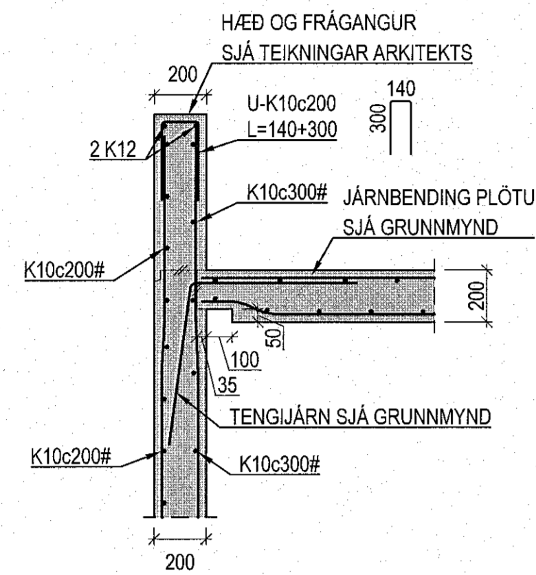
DÆMIGERT SNIÐ: TENING PAKPLÖTU VID ÚTVEGGI 1:20
