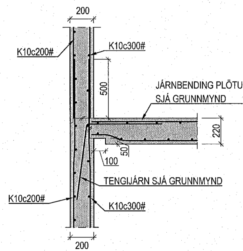
DÆMIGERT SNIÐ: TENING MILLIPLÖTU VID ÚTVEGGI 1:20
