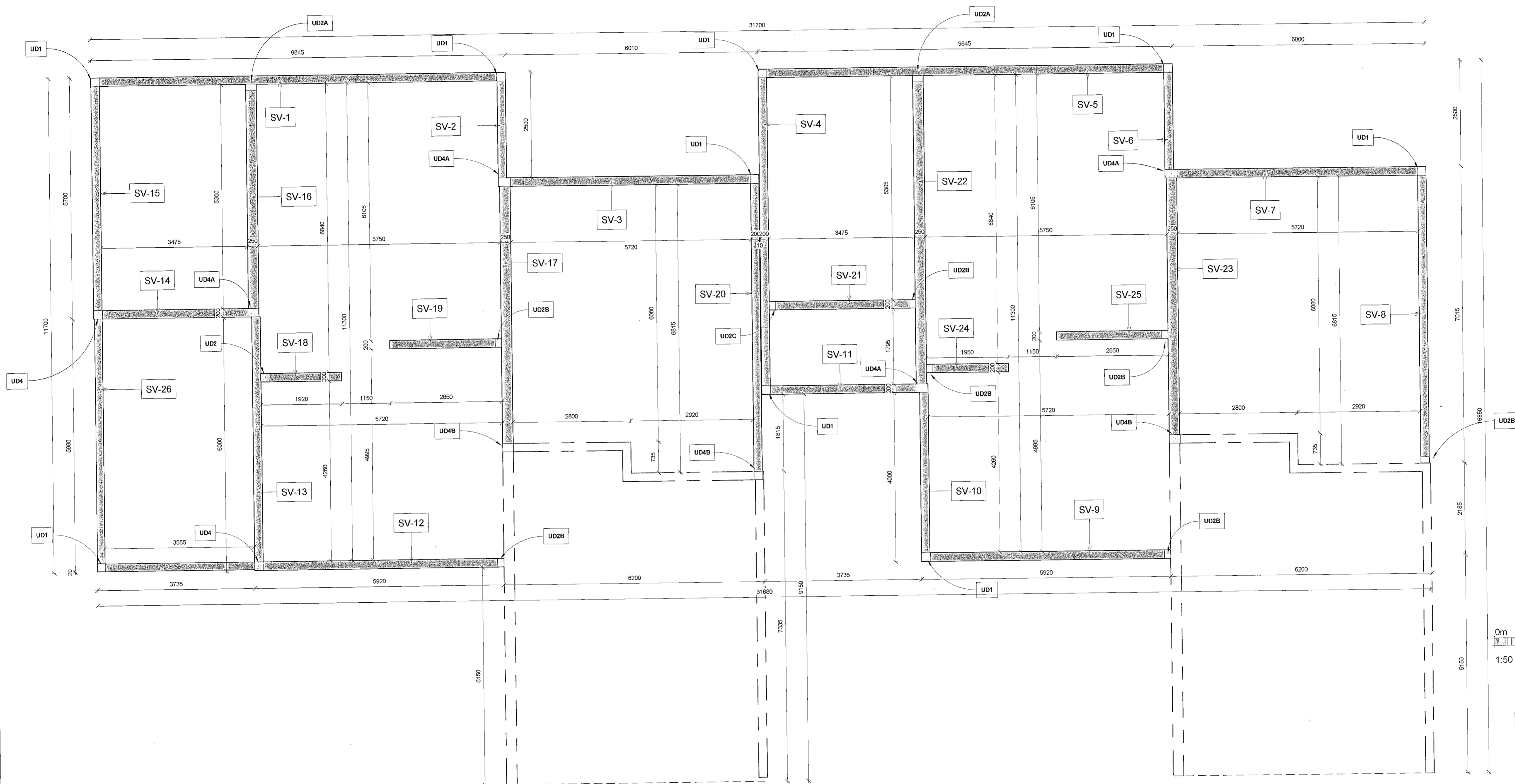
1 Eingar Sökkulveggur 1. Hæð 1 : 50
