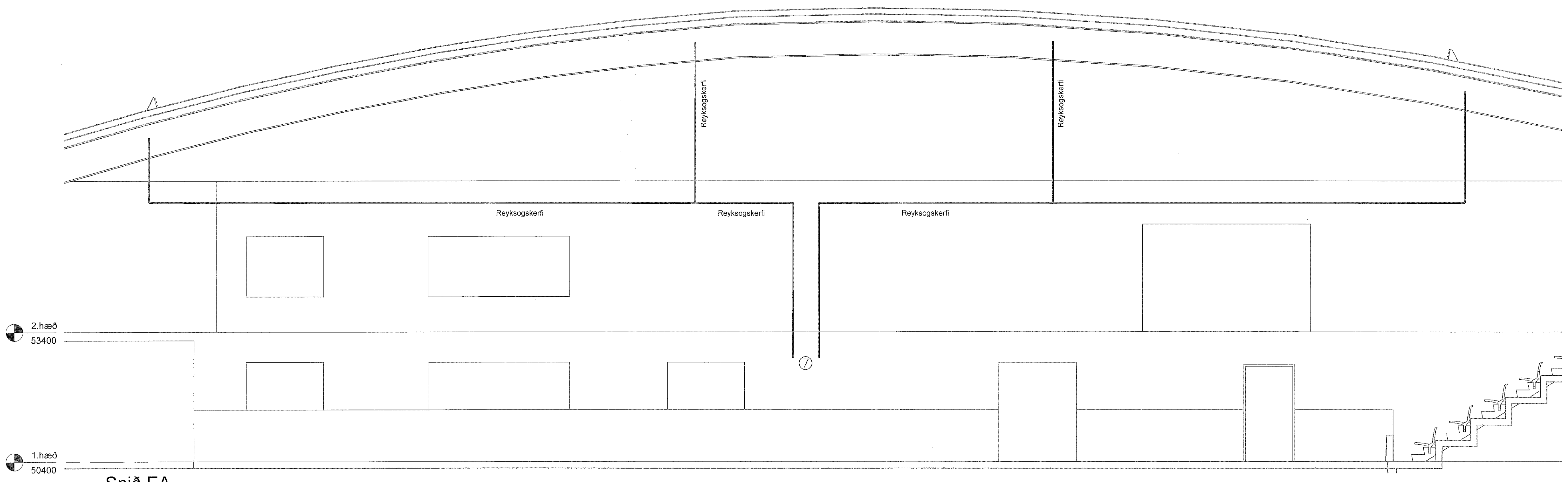
EA Snið EA 01_3_34_03 1 : 50
