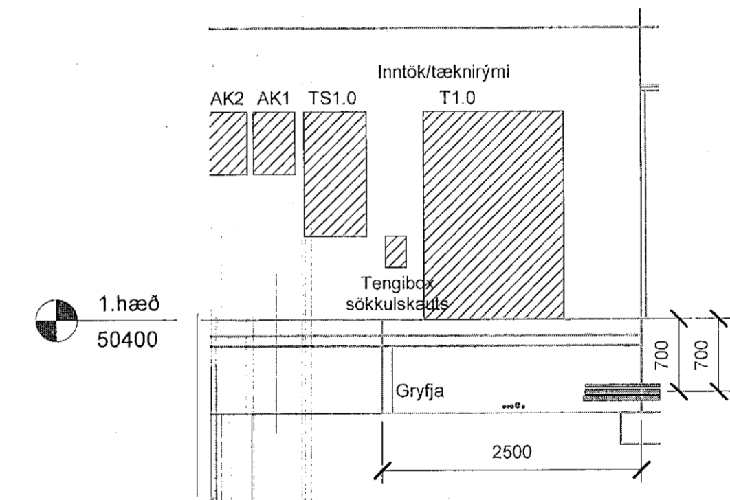
AB Snið AB xx_3_03_01 1:50
