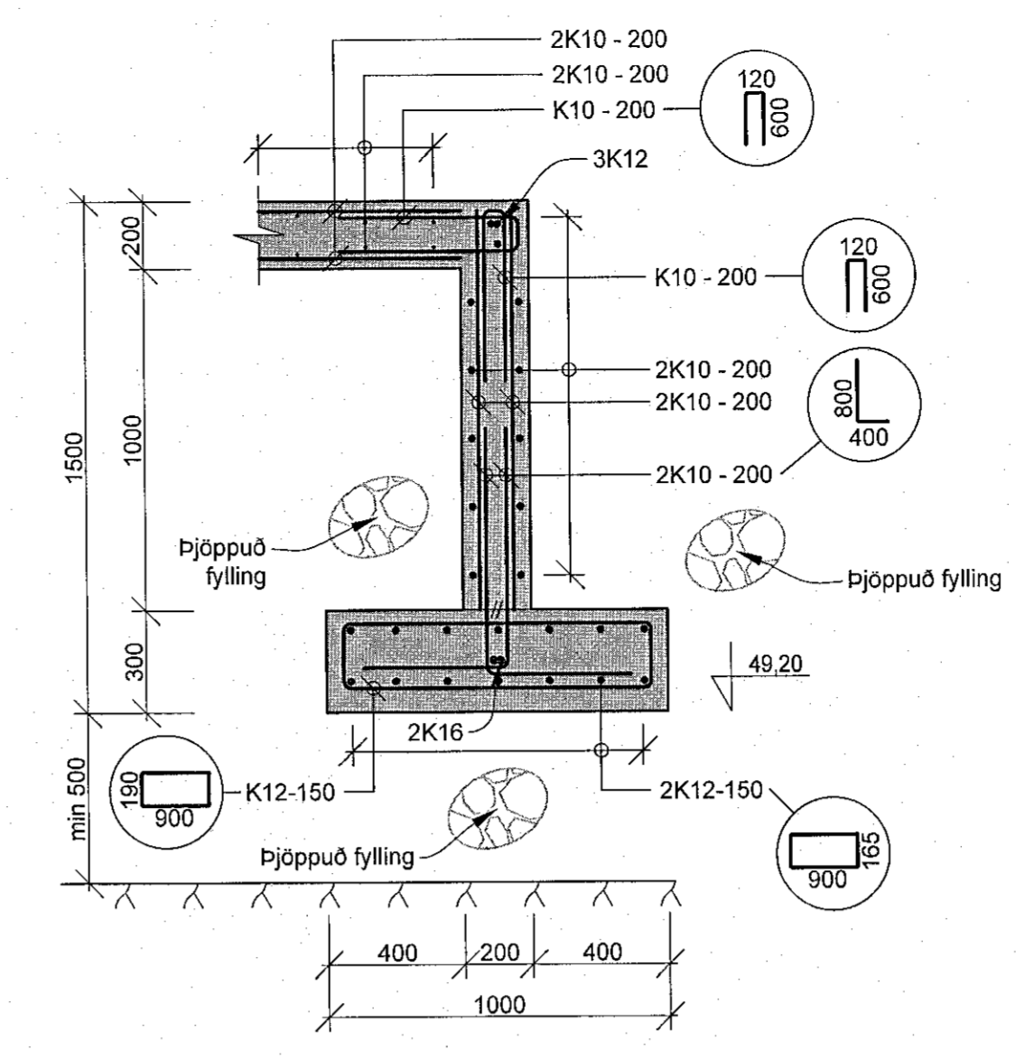
AU Snið 8.G.-1 M 1:20
