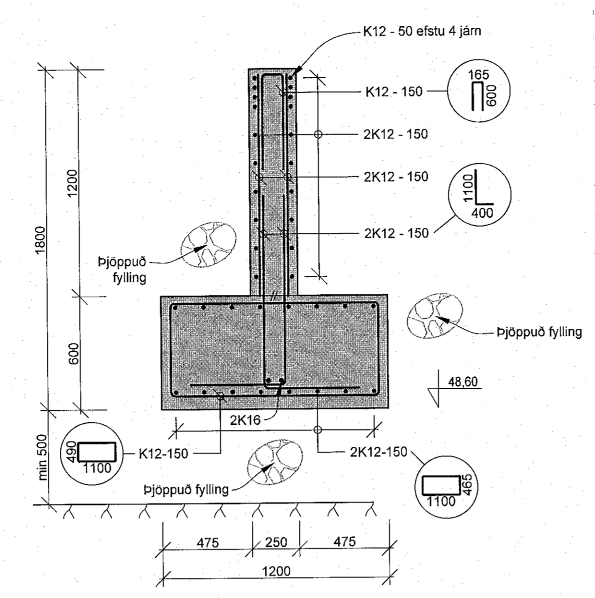
AT Snið 8.G.-1 M 1:20
