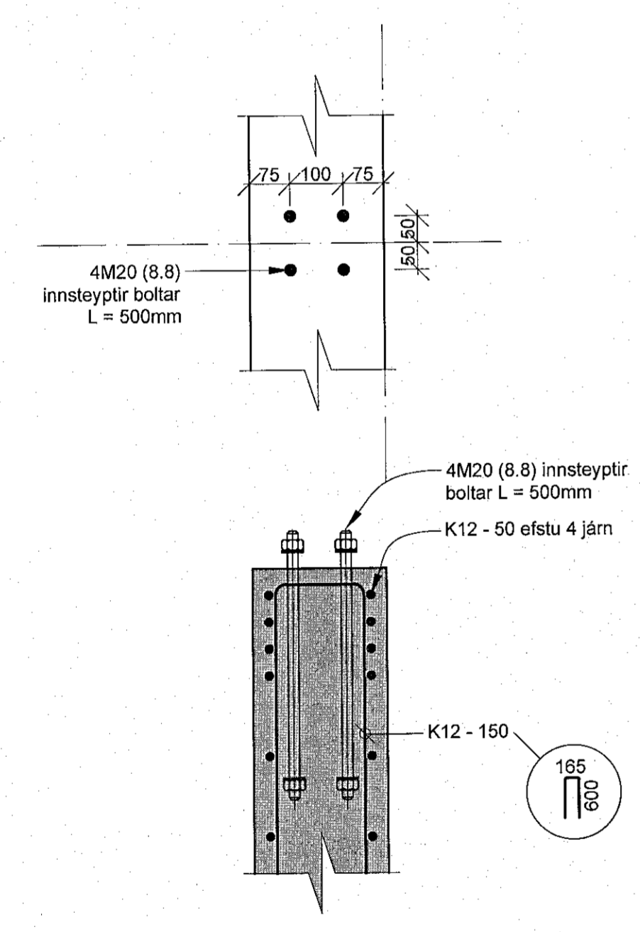
AV Deili/snið 8.G.-1 M 1:20
