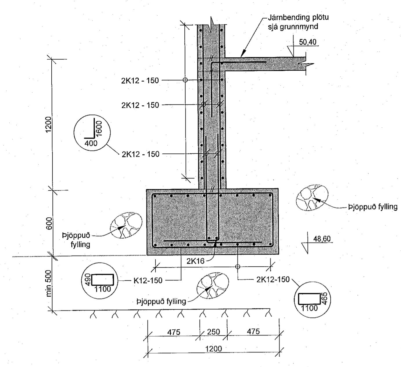
AS Snið 8.G.-1 M 1:20
