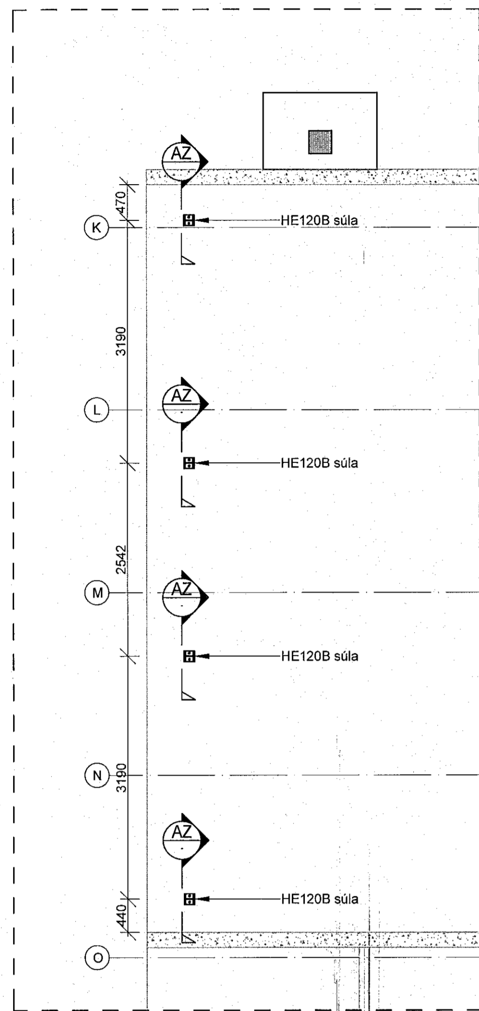
Grunnmynd - Innkeyrsluhurðir M 1:50
