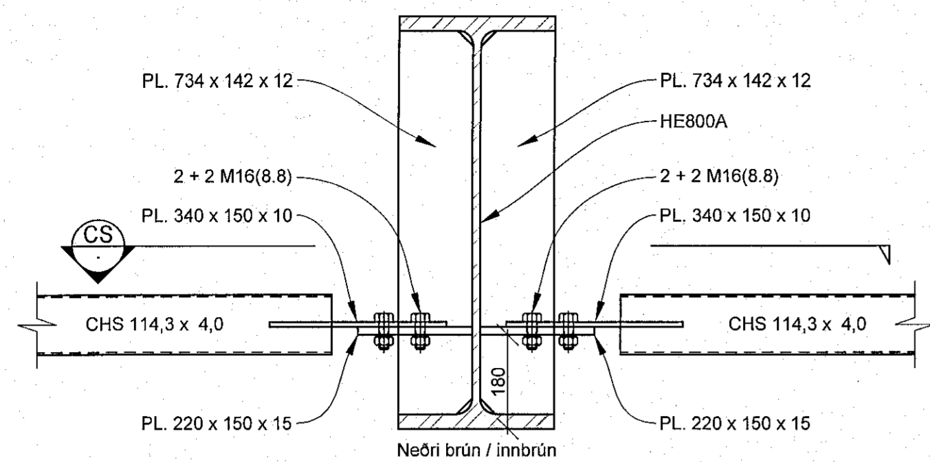
CR Snið M 1:10
