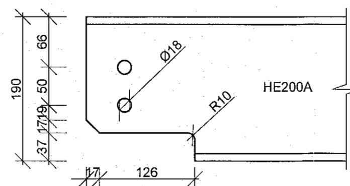
Bitaðendi - HE200A M 1:5
