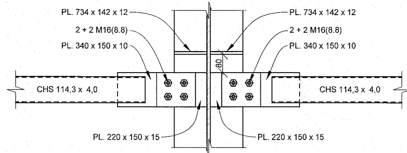
CS Snið M 1:10
