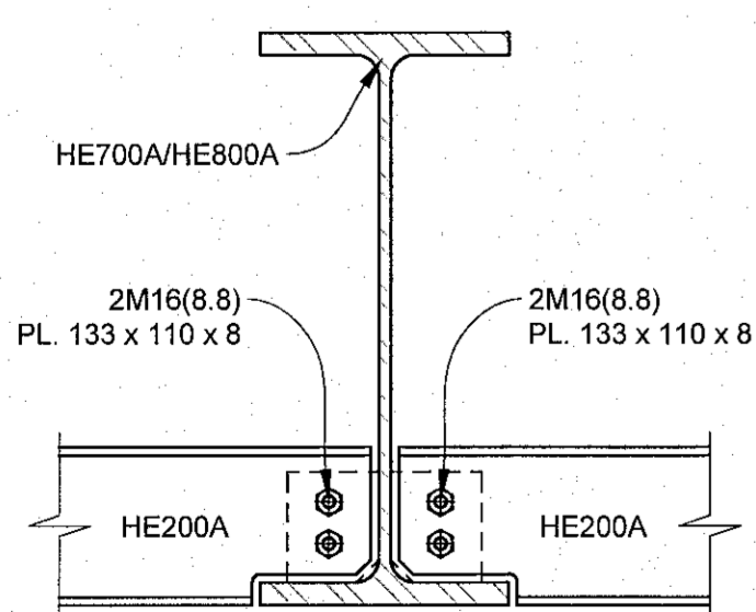
CQ Snið B.S.02 M 1:10
