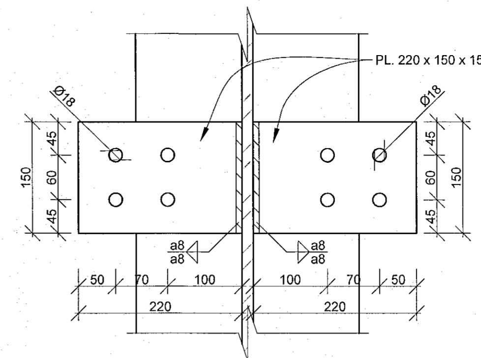
PL. 220 x 150 x 15 M 1:5
