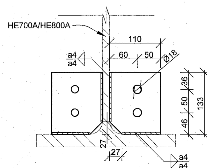
PL. 133 x 110 x 8 M 1:5
